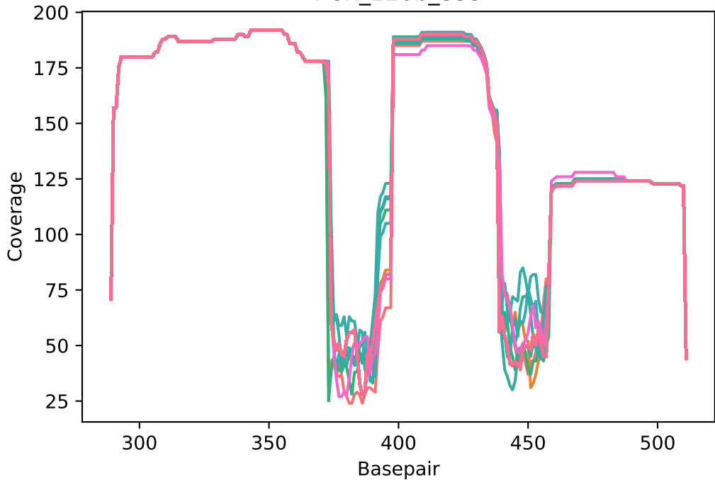
PCR_220b_S33
