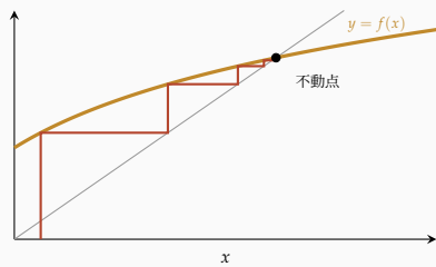
クモの巣図：不動点の近くで f が増加かつ 0 < f' < 1 \Rightarrow 単調収束。
