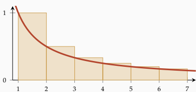
上側和と積分の比較： \ln(n+1) < H_n < 1 + \ln n 。同じ図で積分判定法のあらゆる評価が証明できる。
