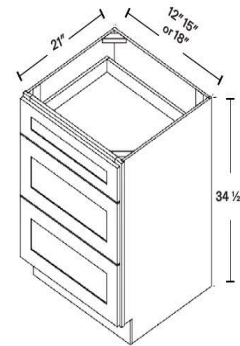
VANITY DRAWER BASE VANITÉ AVEC TIROIRS
