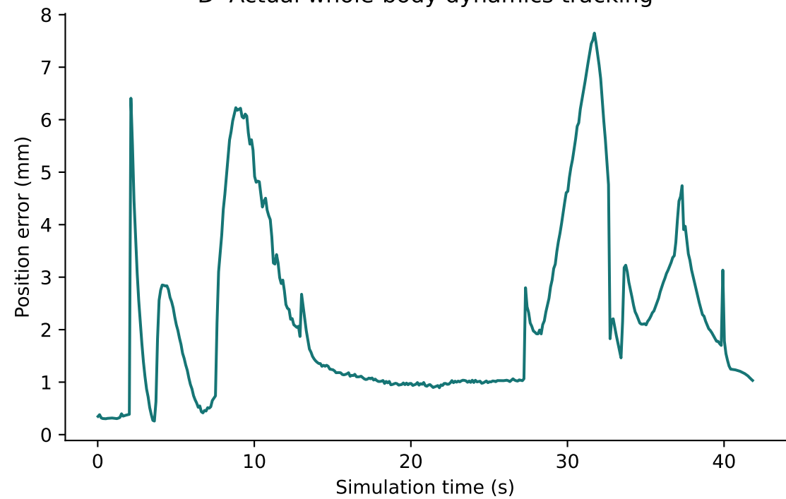
D Actual whole-body dynamics tracking
