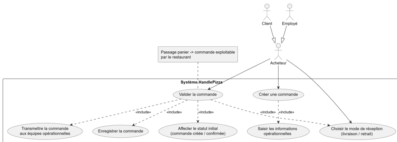
Diagramme de cas d'utilisation de gestion de la commande client
