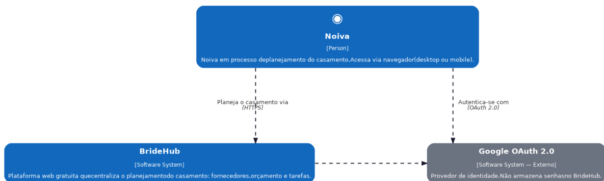
Diagrama de Contexto — BrideHub Nível 1 · Modelo C4 · Engenharia de Software — Católica SC
