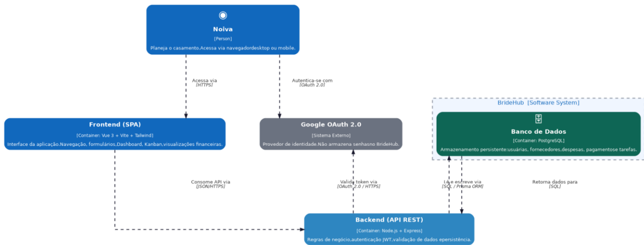
Diagrama de Containers — BrideHub Nível 2 : Modelo C4 - Engenharia de Software — Católica SC
