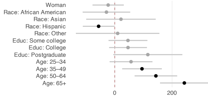
Keylogging
