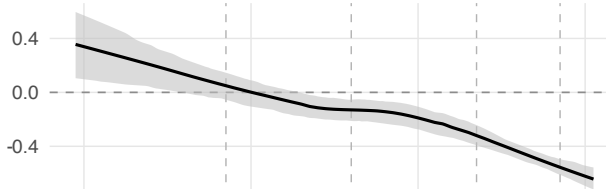
Facebook Pixel
