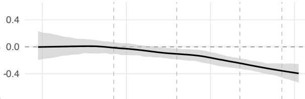
Keylogging
