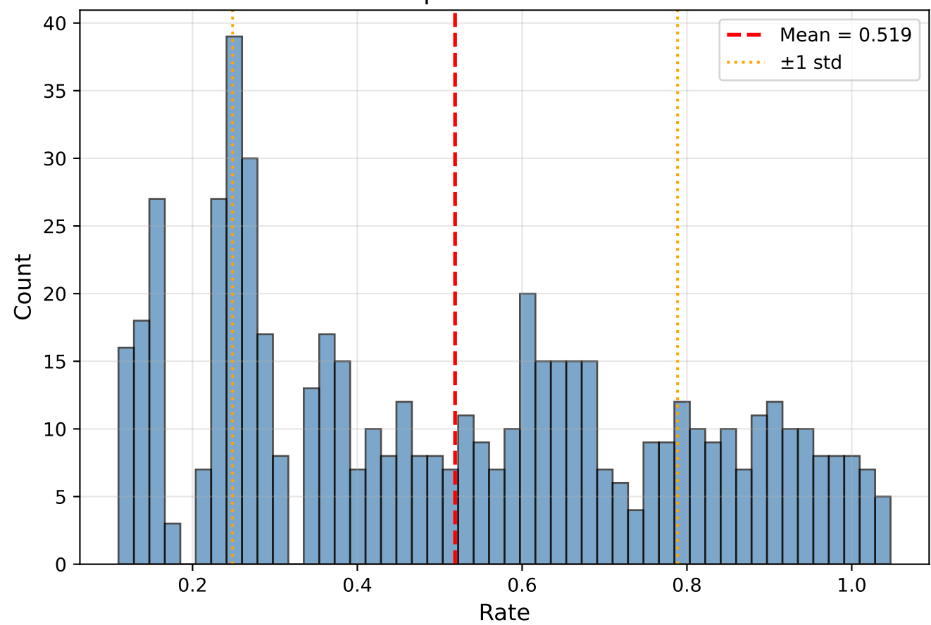
Epistasis = 0.7
