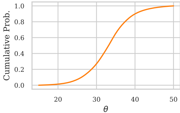
Posterior CDF
