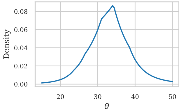
Posterior PDF
