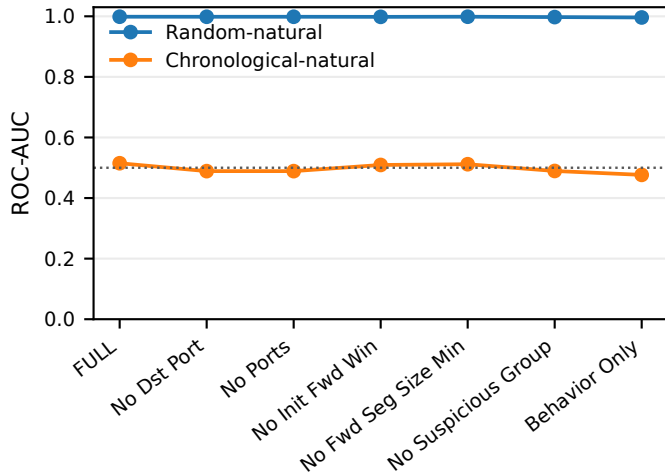
(b) ROC-AUC
