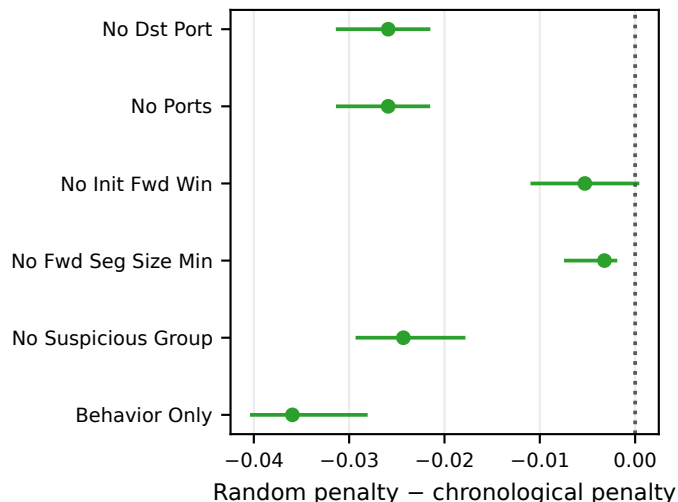
(d) ROC-AUC shortcut interaction
