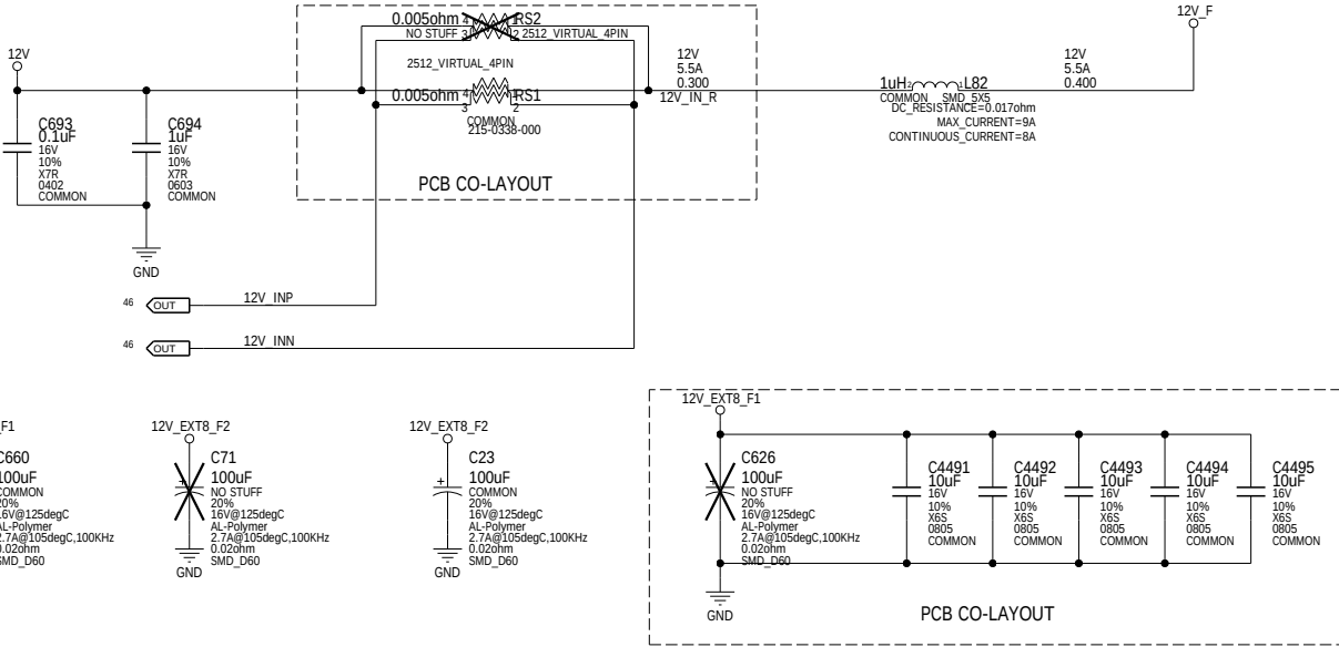
PEX_12V INPUT - 66W
