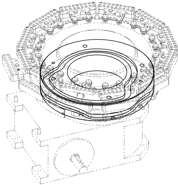
Stückliste: 8-104-322-014
