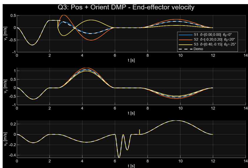
Figure 12: Γραμμικές ταχύτητες τελικού οργάνου (Ερώτημα 3).
