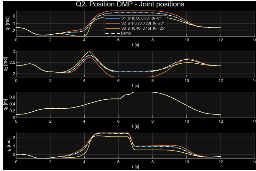
Figure 9: Θέσεις αρθρώσεων \mathbf{q}(t) (Ερώτημα 2).
