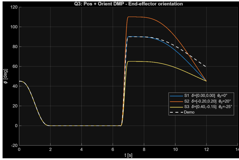
Figure 13: Προσανατολισμός \phi τελικού οργάνου με χρήση DMP (Ερώτημα 3).
