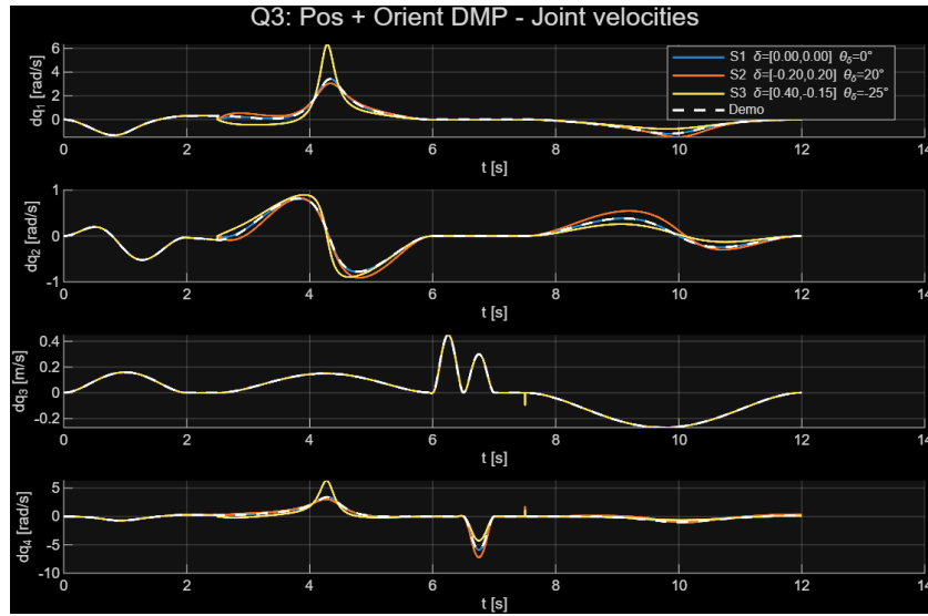
Figure 15: Ταχύτητες αρθρώσεων \dot{\mathbf{q}}(t) (Ερώτημα 3).
