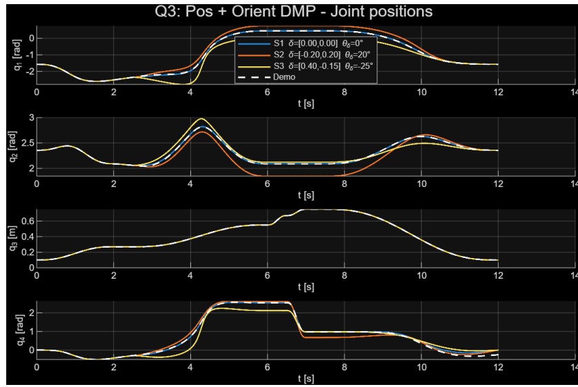
Figure 14: Θέσεις αρθρώσεων \mathbf{q}(t) (Ερώτημα 3).
