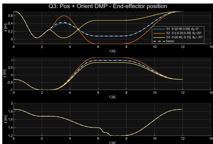
Figure 11: Θέση τελικού οργάνου ( x, y, z ) με πλήρη προσαρμογή (Ερώτημα 3).
