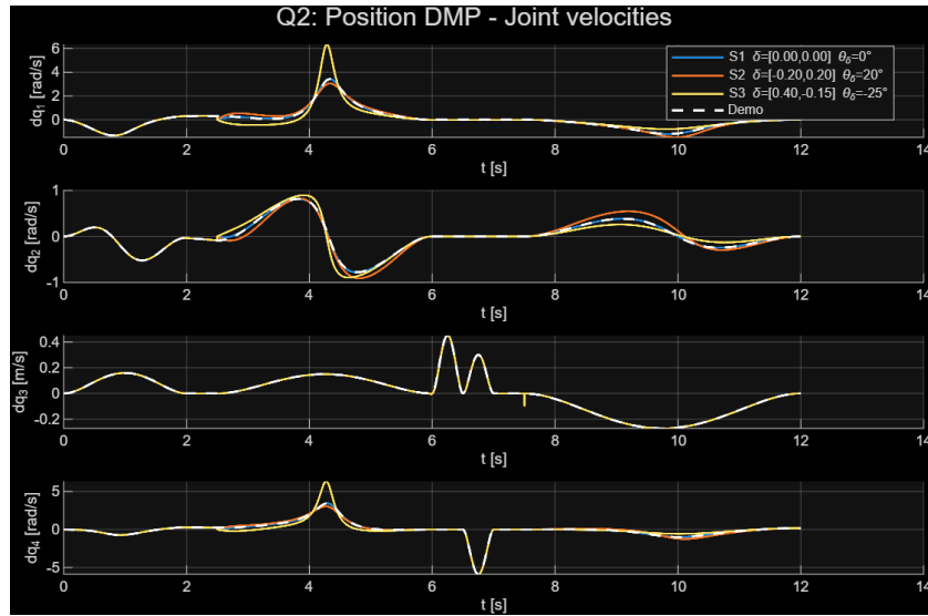
Figure 10: Ταχύτητες αρθρώσεων \dot{\mathbf{q}}(t) (Ερώτημα 2).
