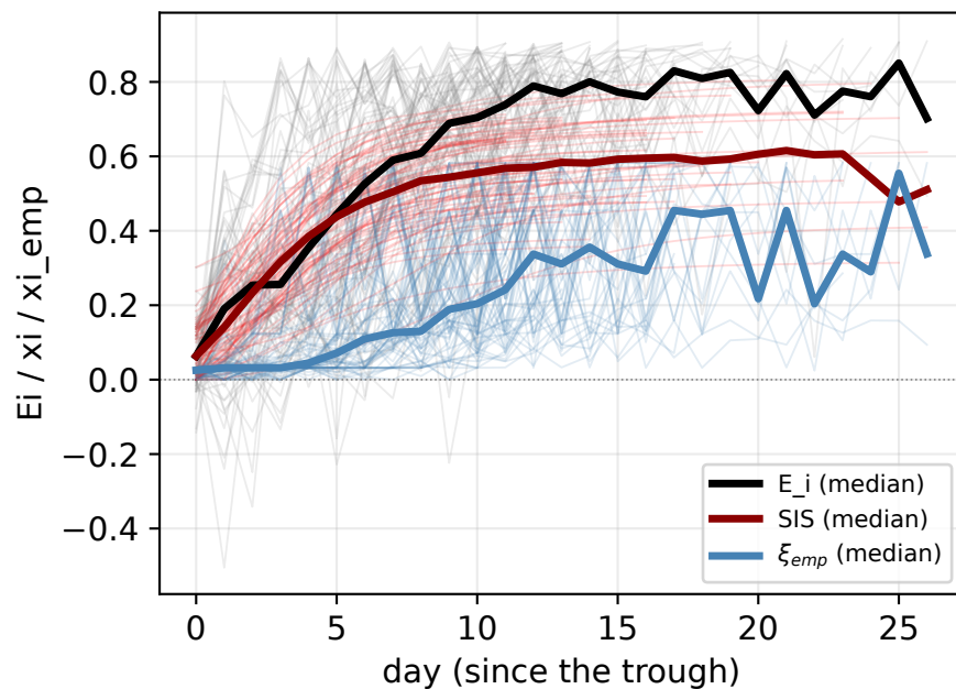
VAR(1) (n=71)
