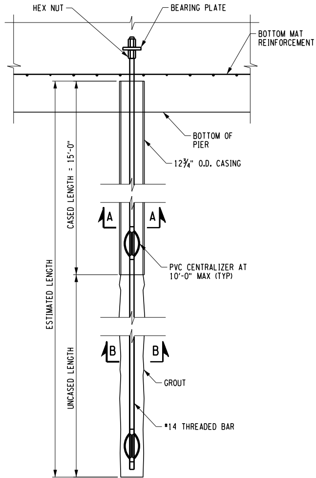
TYPICAL MICROPILE ELEVATION SCALE: N.T.S.
