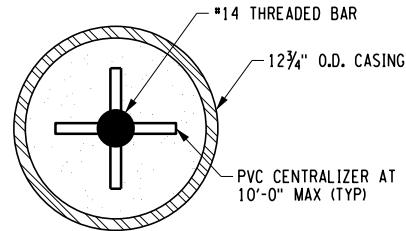
MICROPILE SECTION A-A SCALE: N.T.S.
