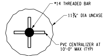
MICROPILE SECTION B-B SCALE: N.T.S.
