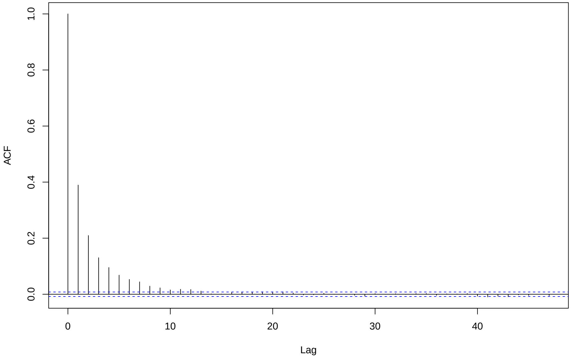
ACF for eta[2,8]
