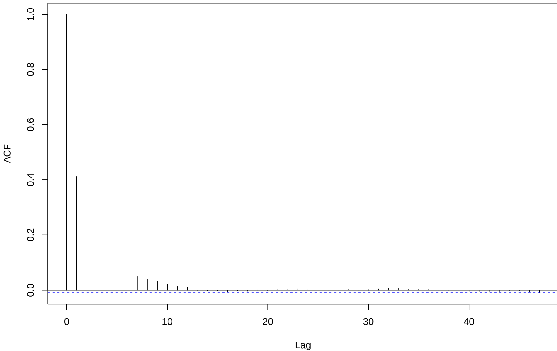
ACF for eta[2,2]
