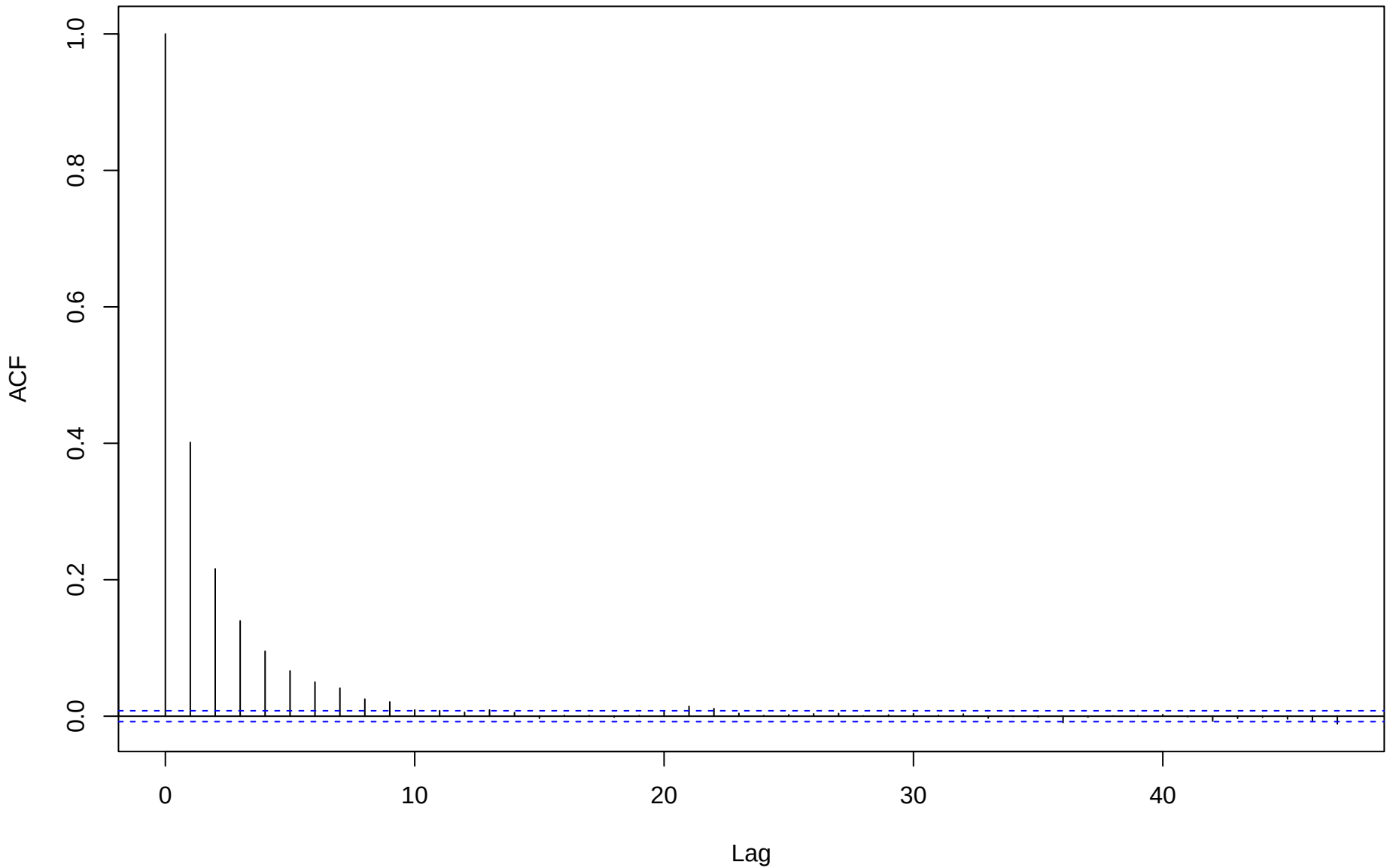
ACF for eta[1,6]
