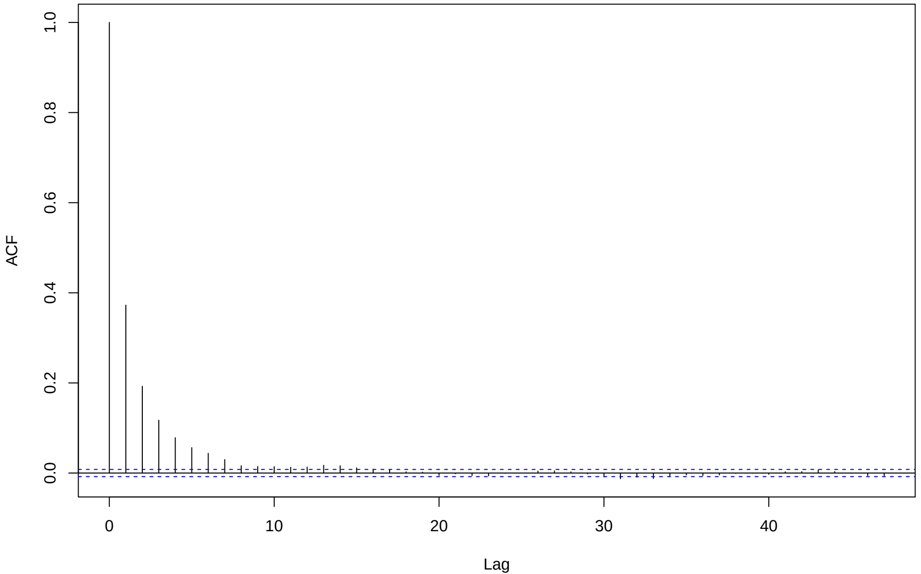
ACF for eta[2,1]
