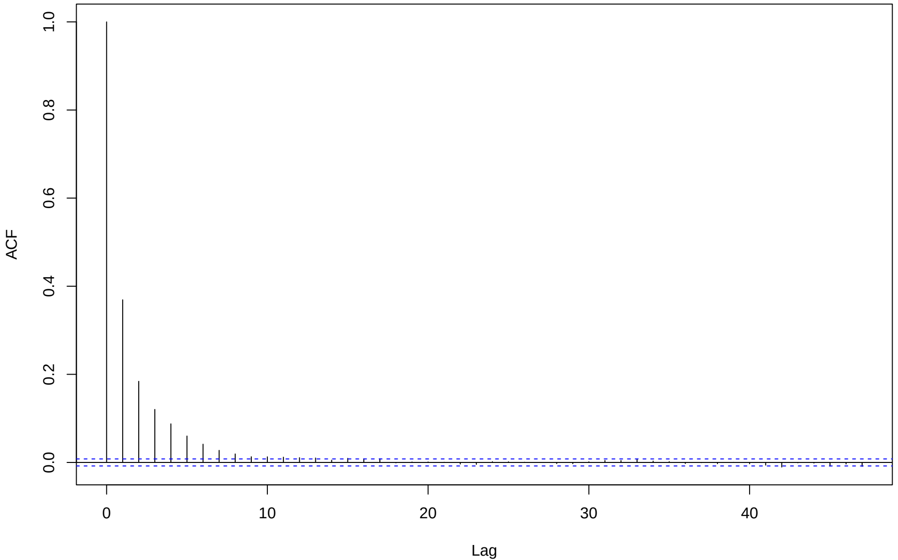
ACF for eta[5,3]
