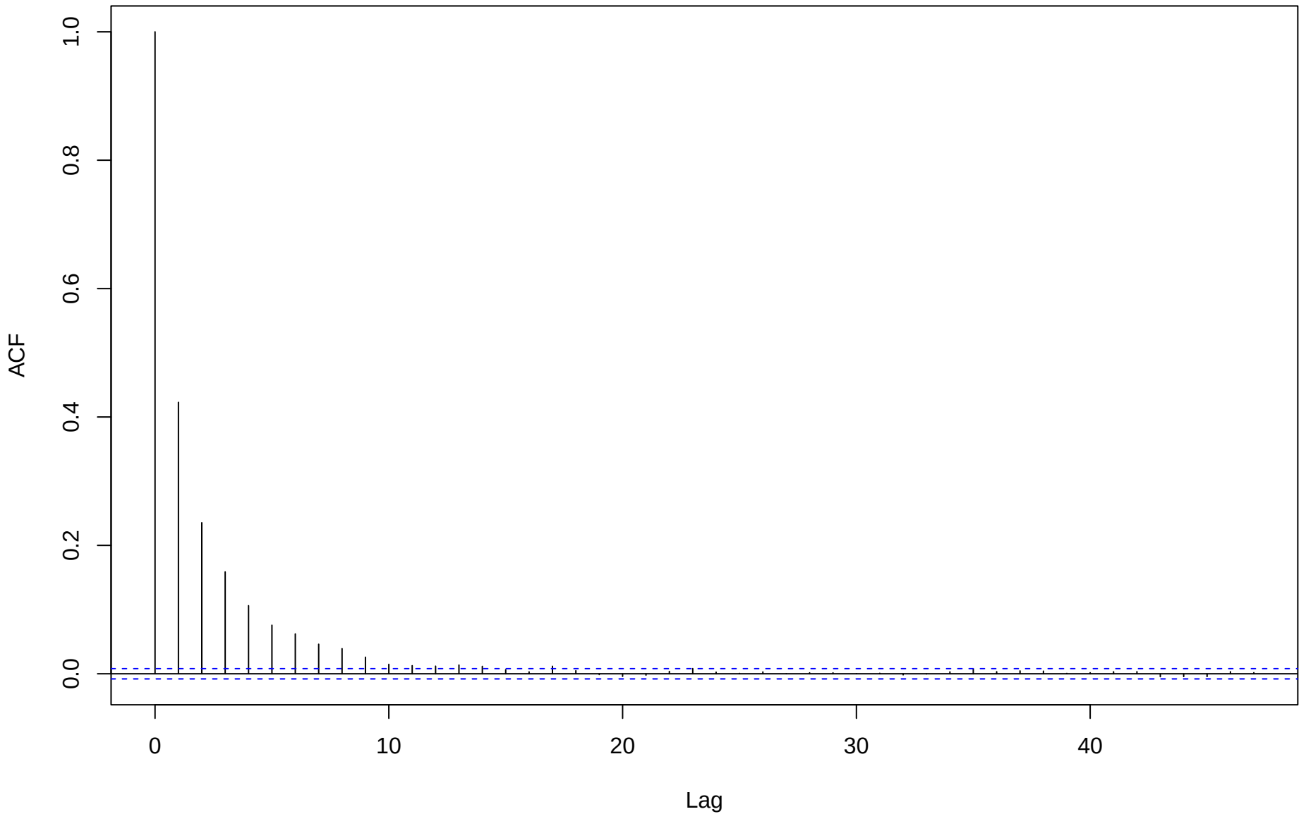
ACF for eta[1,4]
