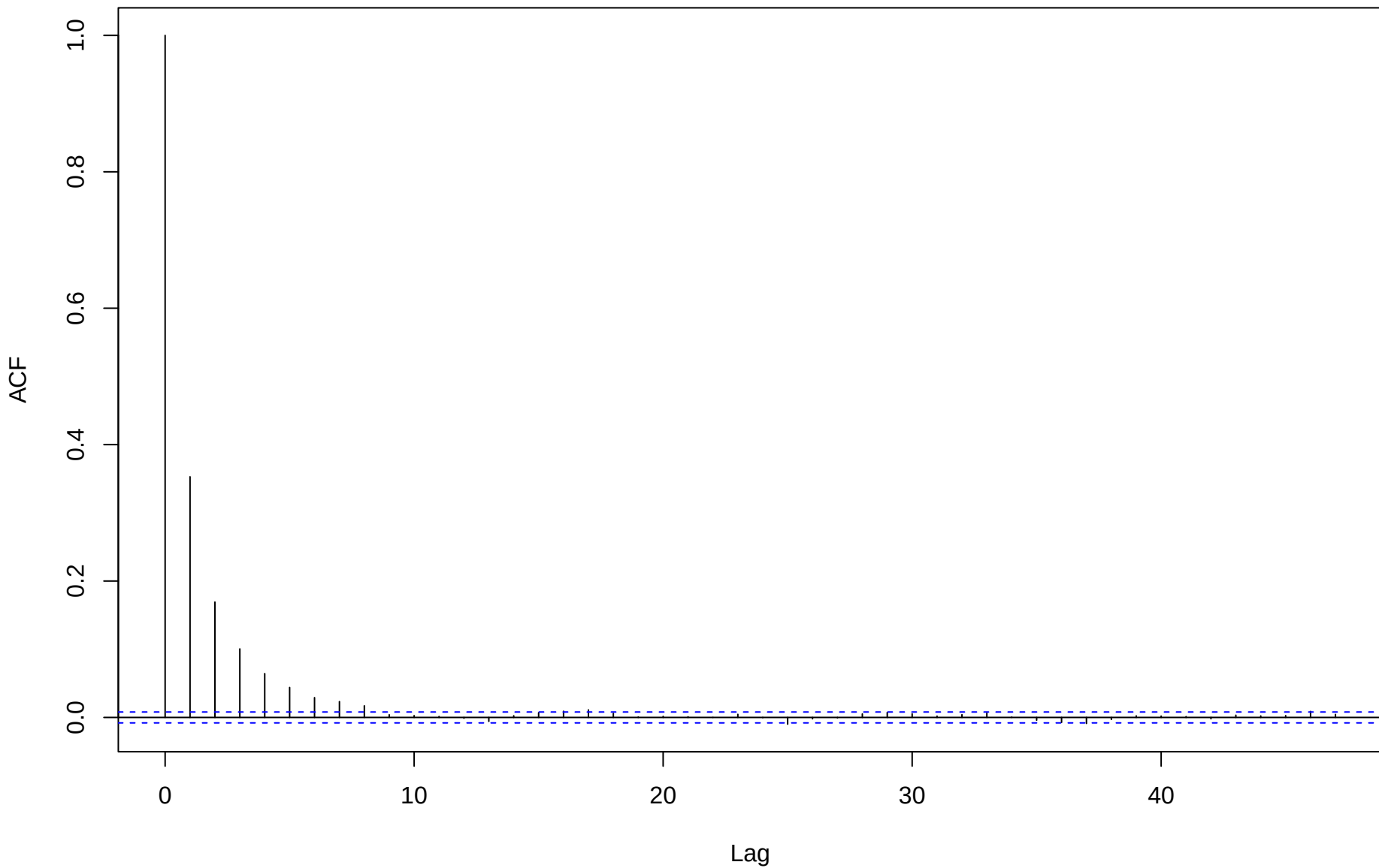
ACF for eta[3,1]
