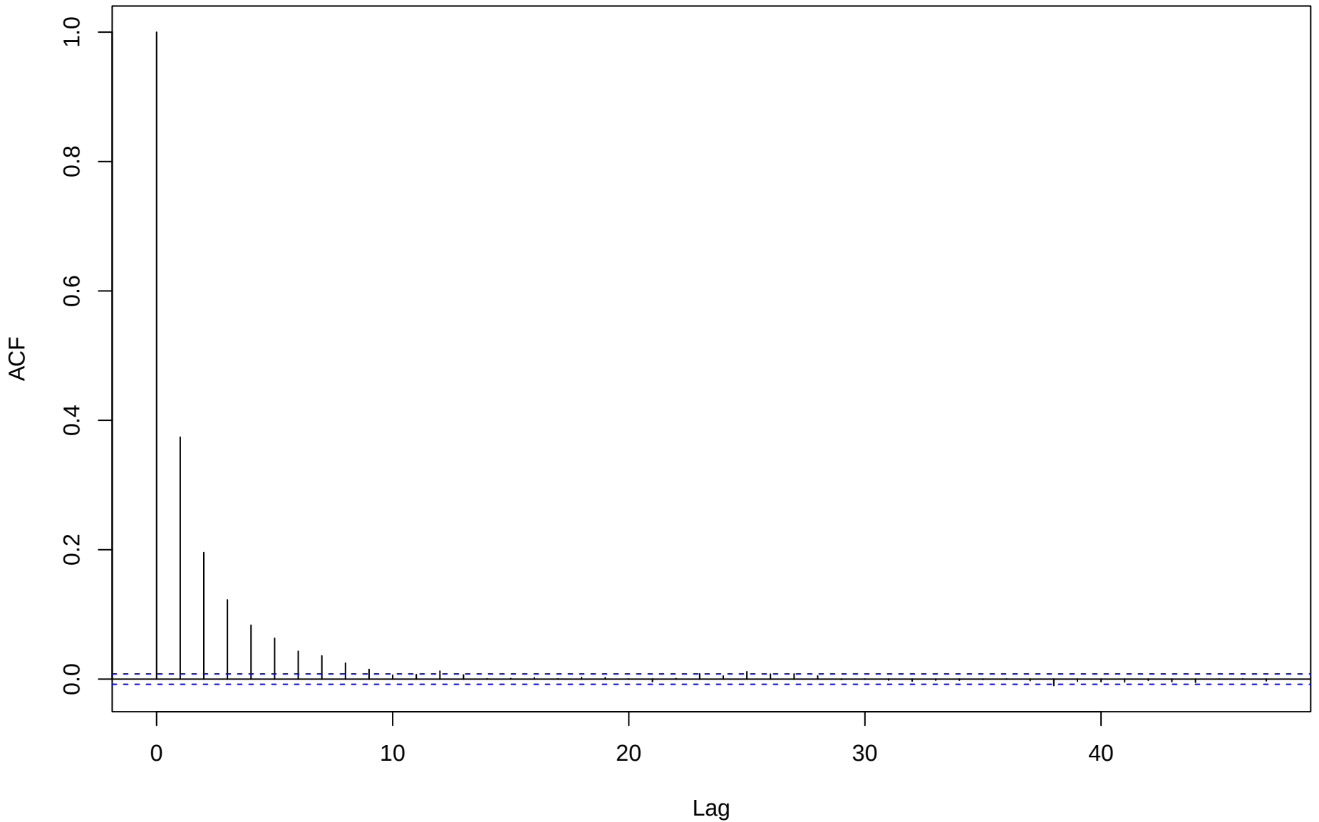
ACF for eta[1,8]
