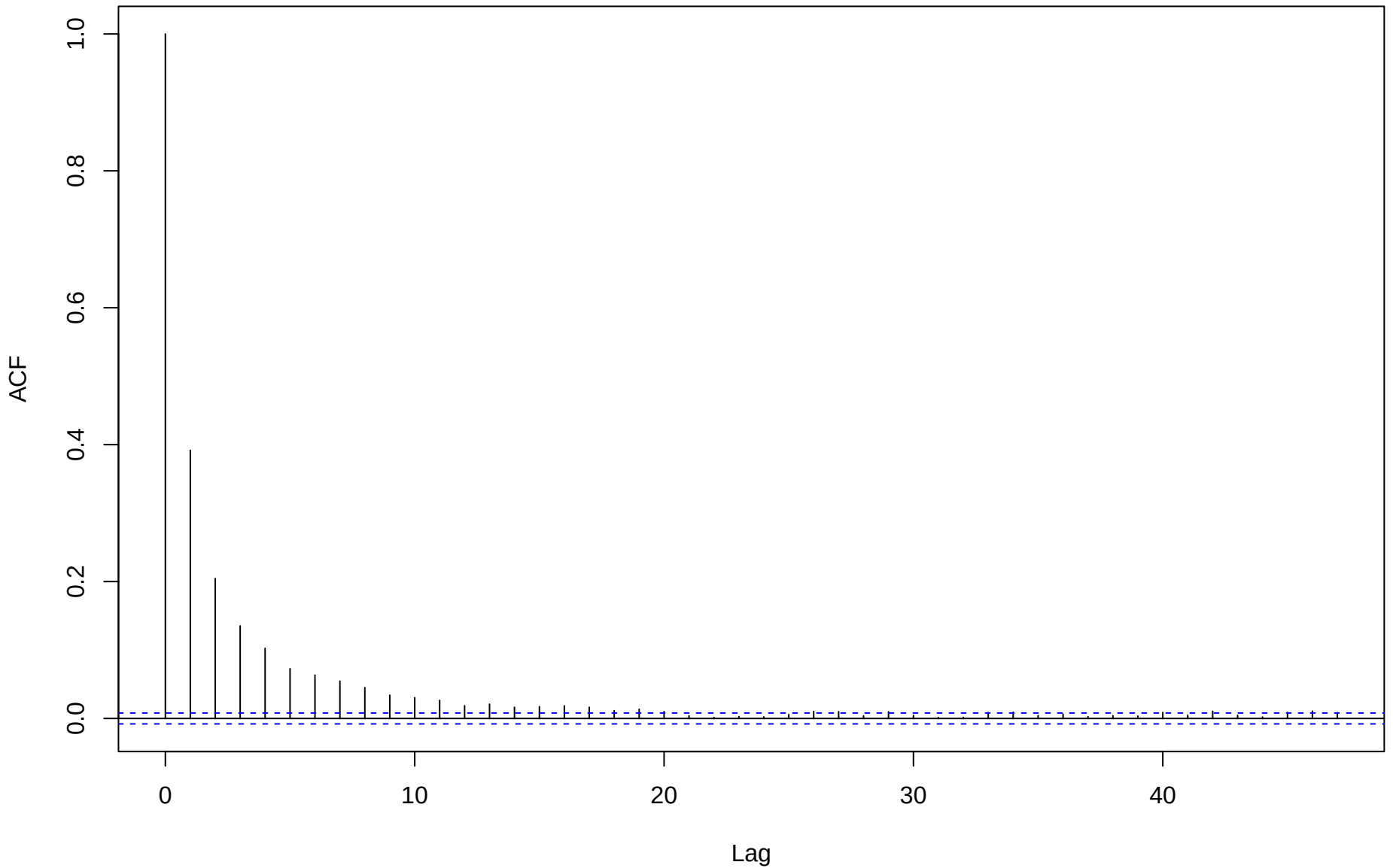
ACF for eta[4,1]
