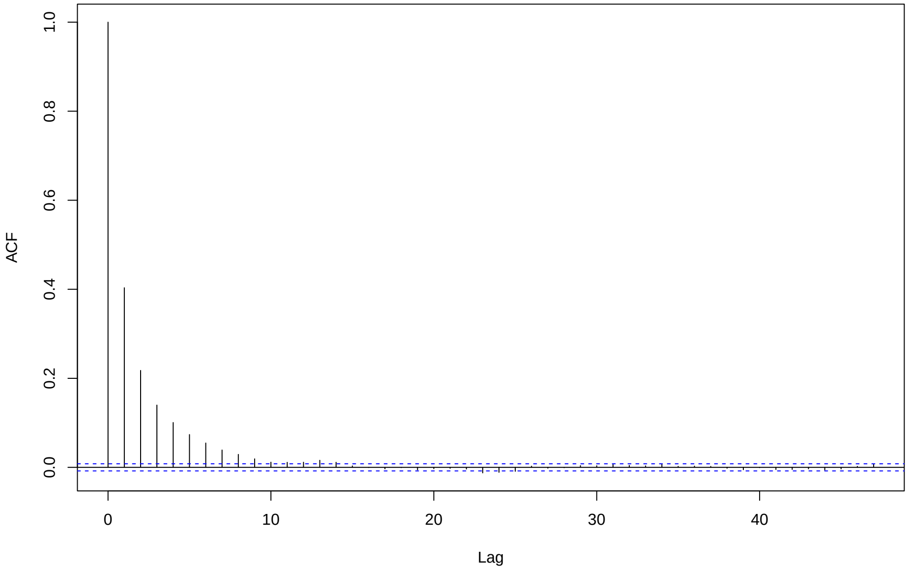
ACF for eta[4,7]
