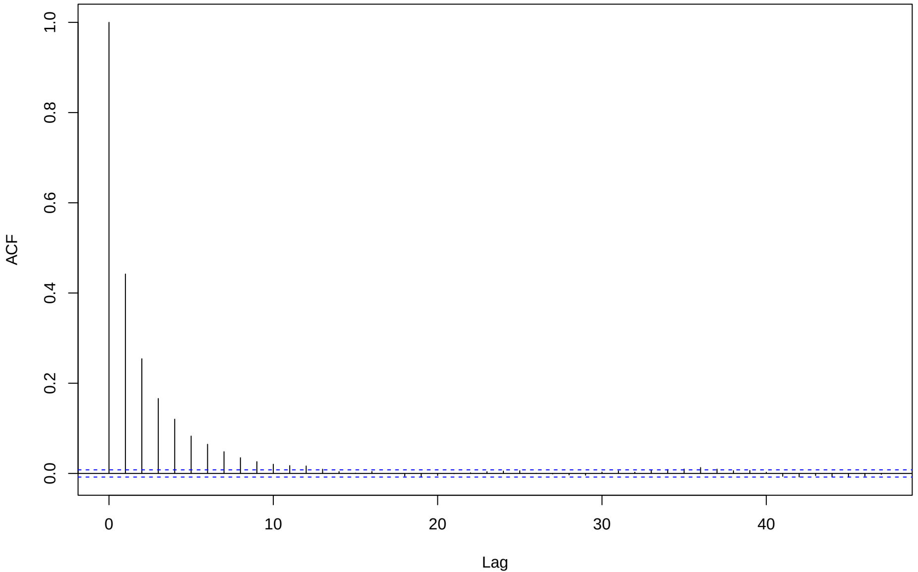
ACF for eta[3,9]
