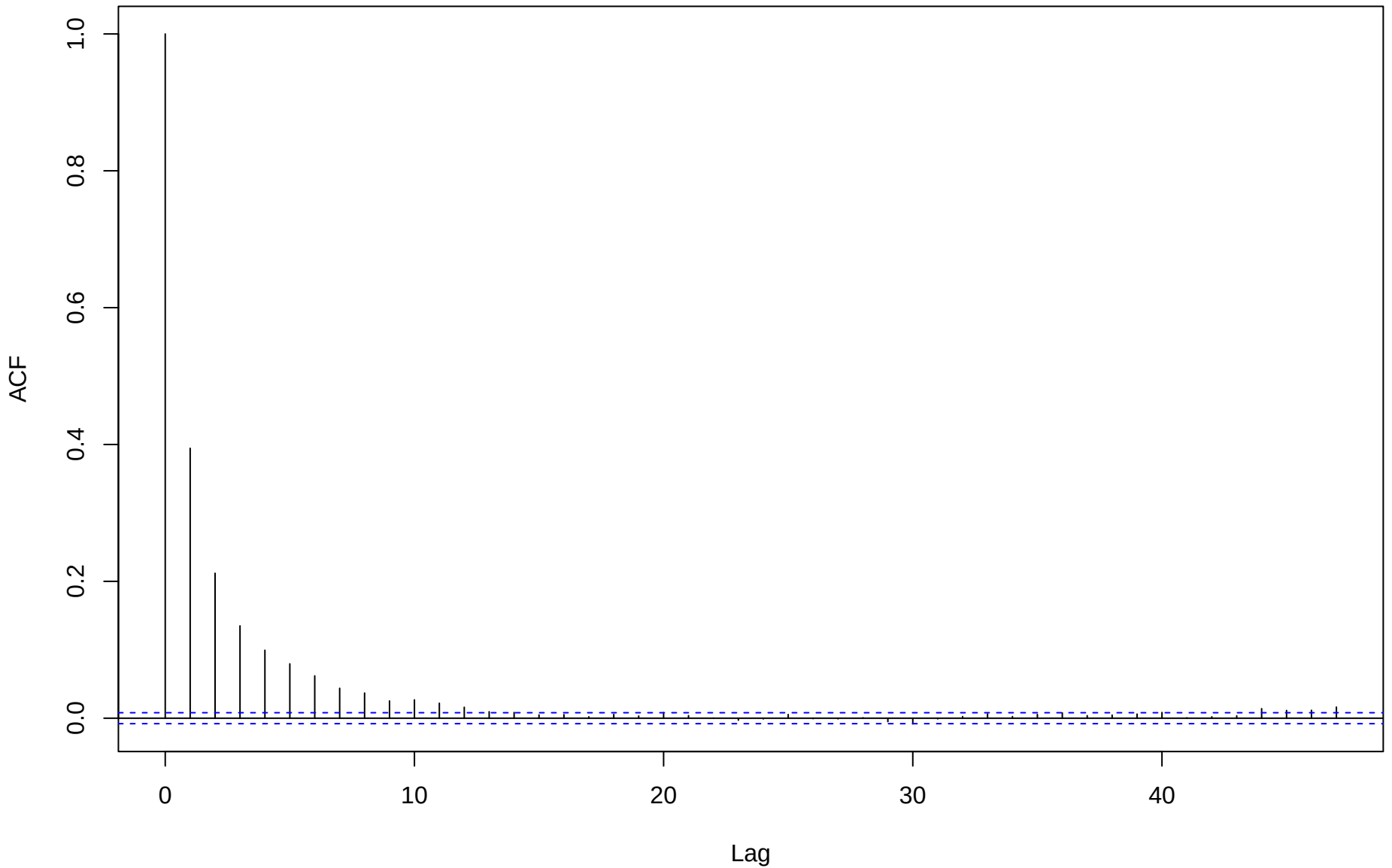
ACF for eta[4,8]
