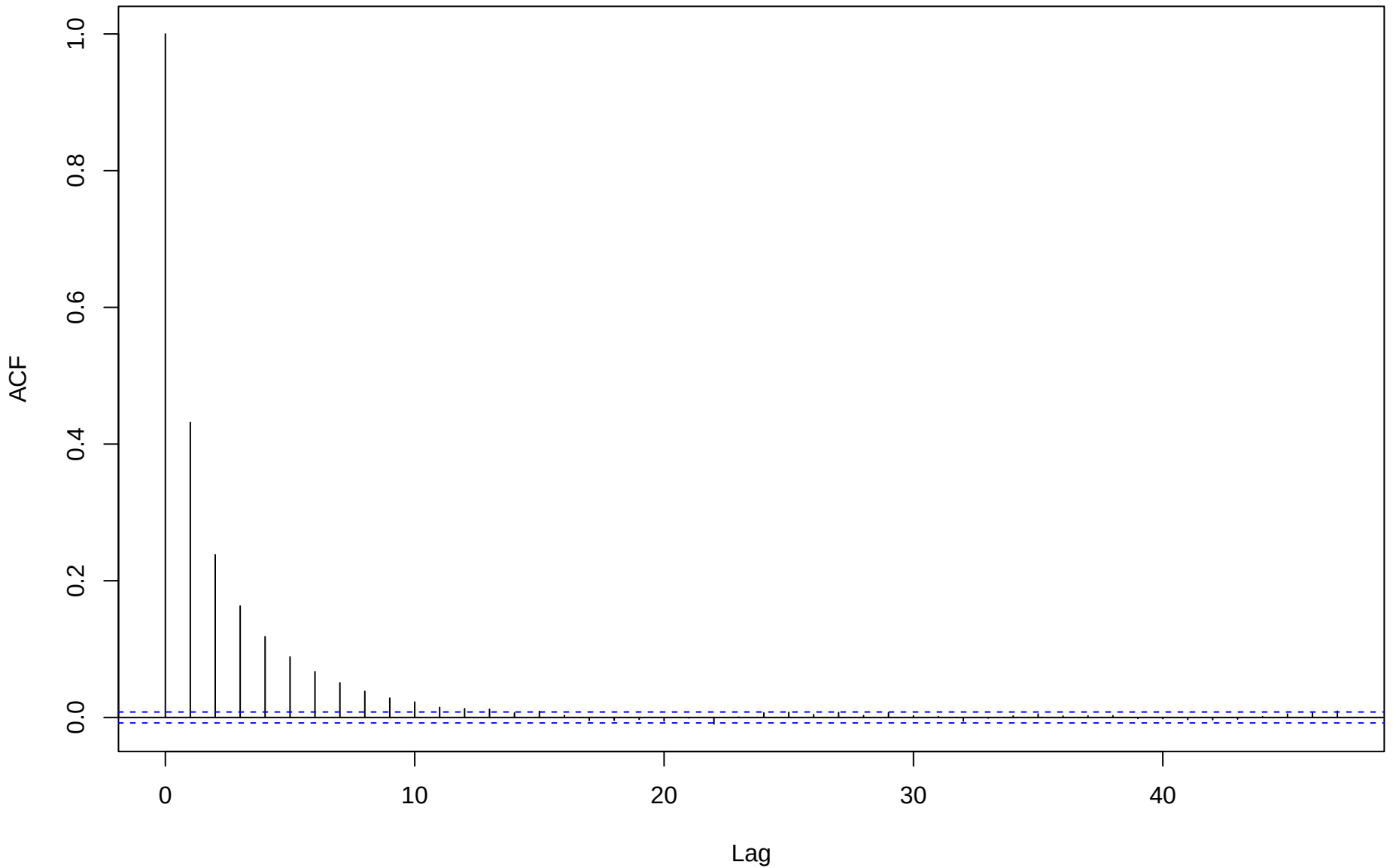
ACF for eta[4,2]
