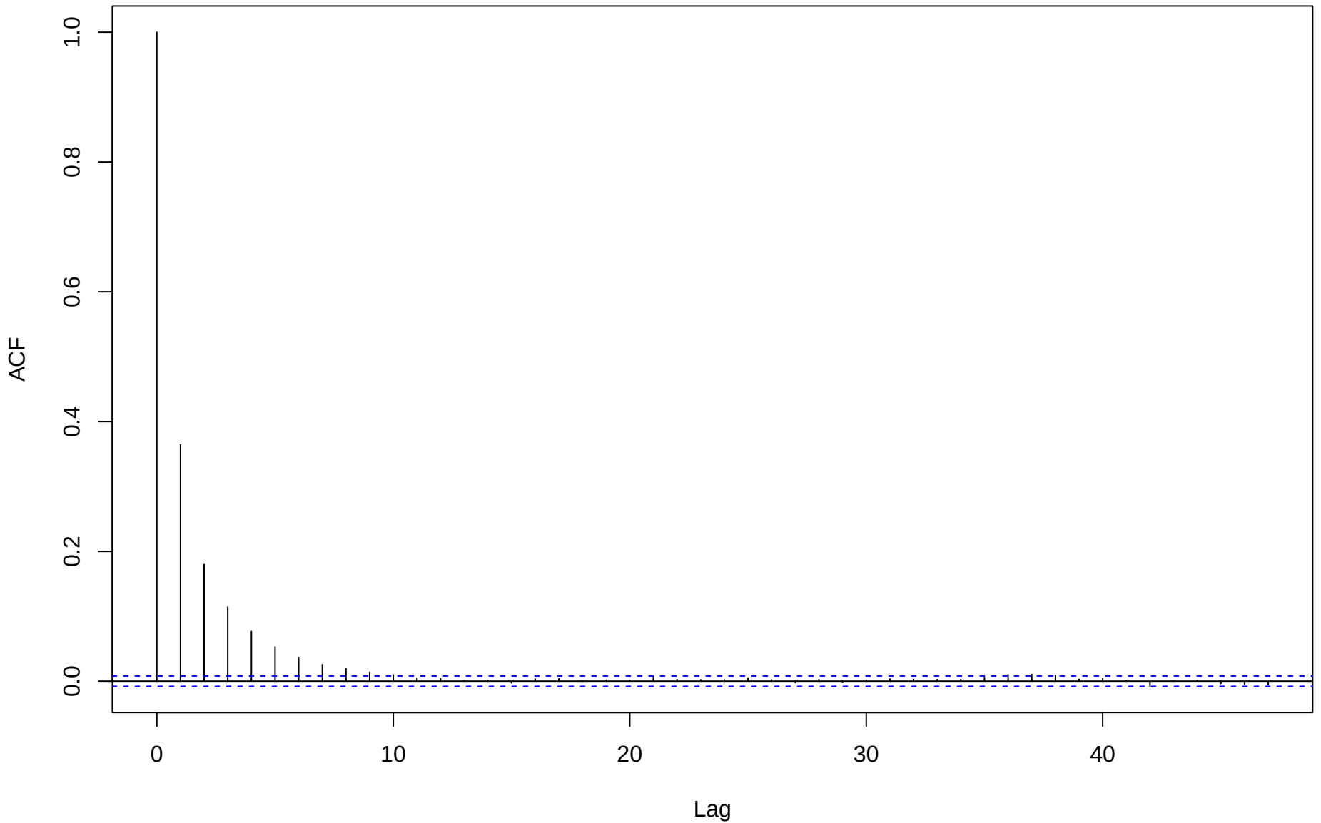
ACF for eta[5,8]
