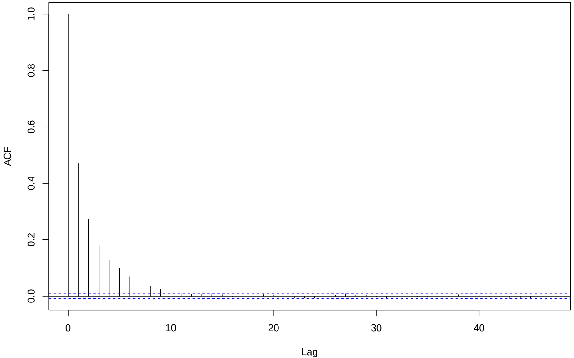
ACF for eta[5,4]
