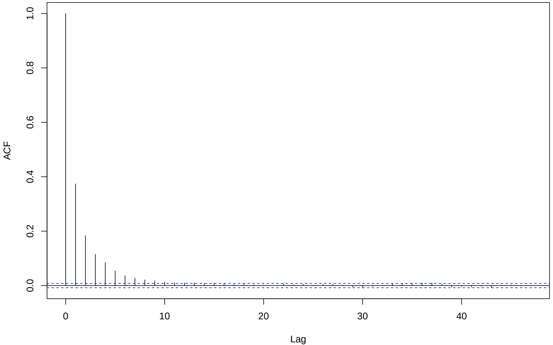
ACF for eta[5,7]
