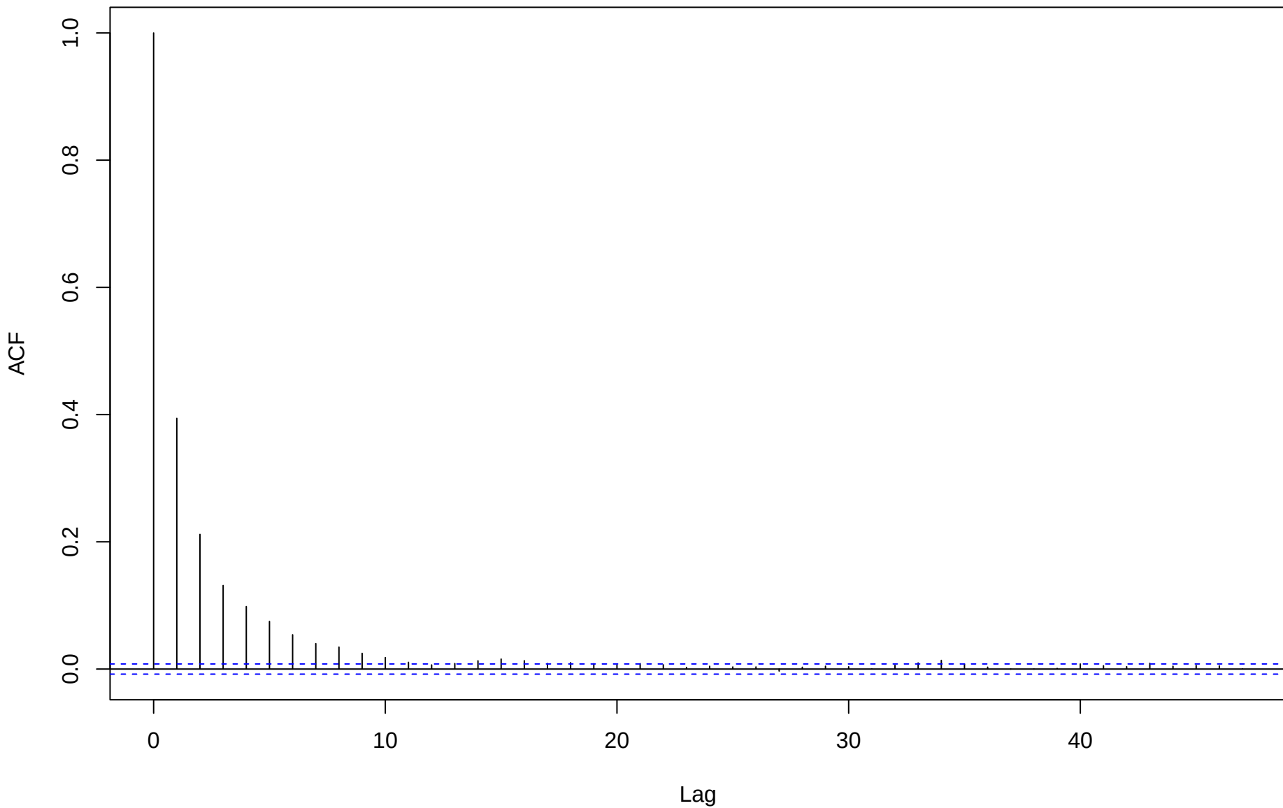
ACF for eta[4,4]
