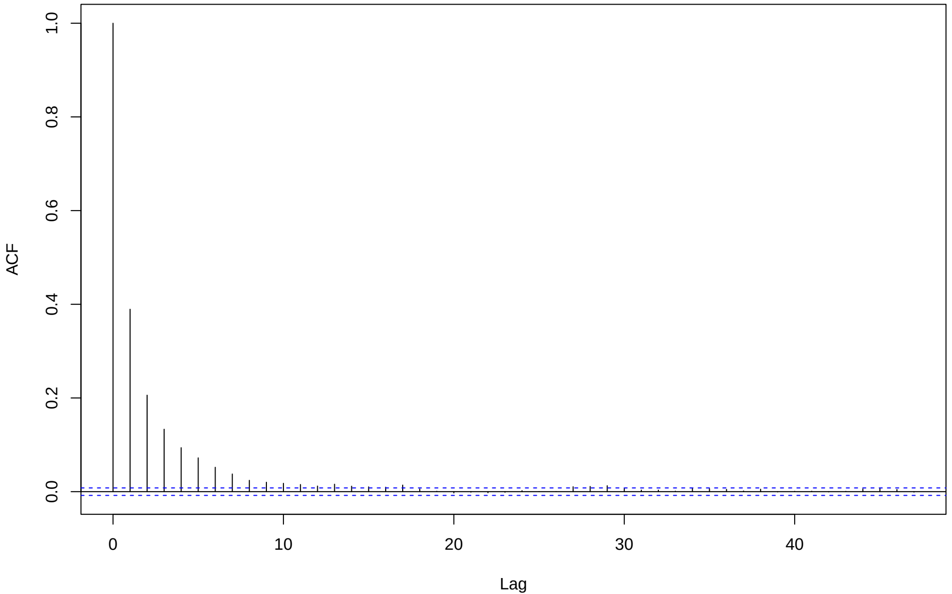
ACF for eta[4,9]
