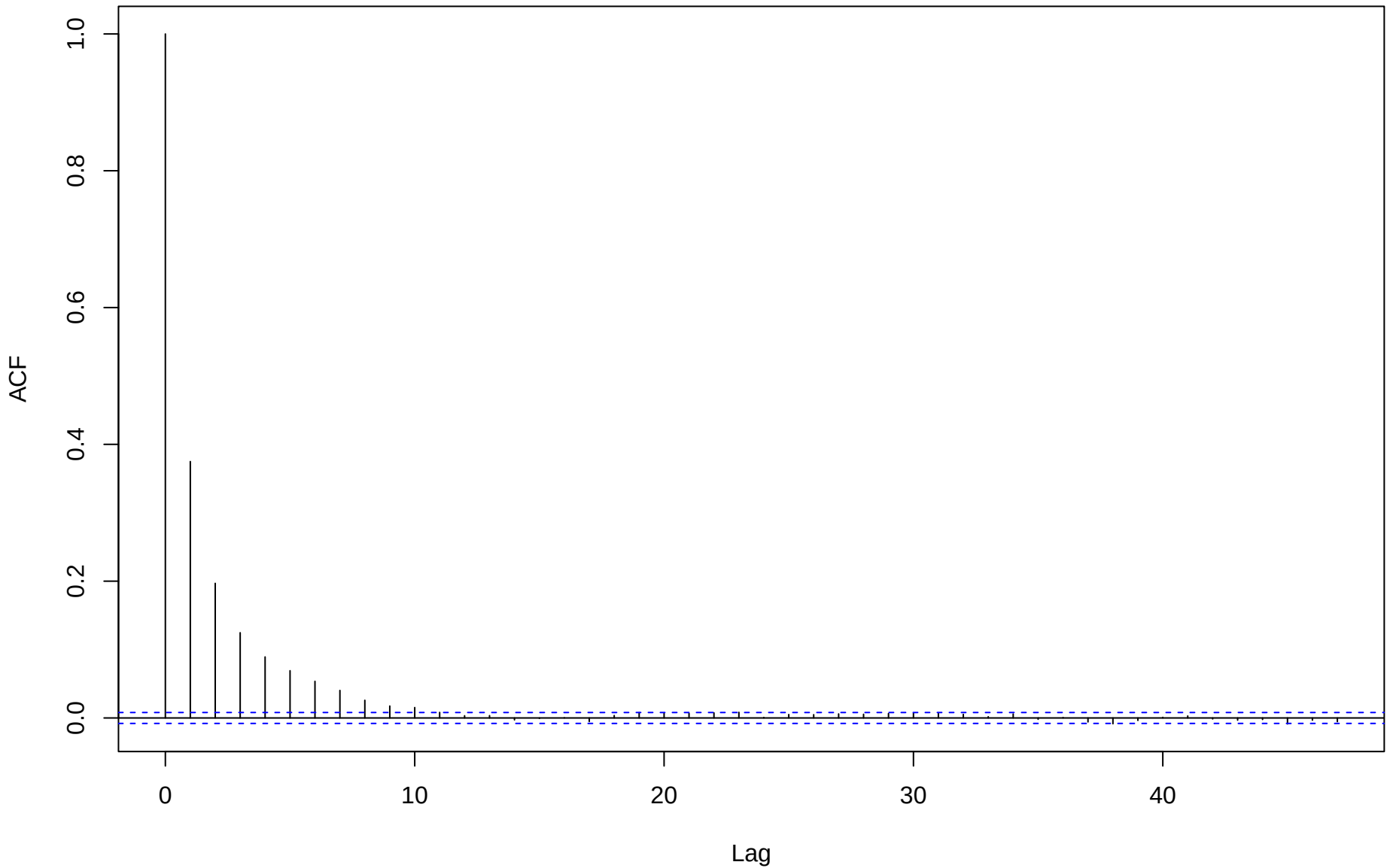
ACF for eta[1,2]
