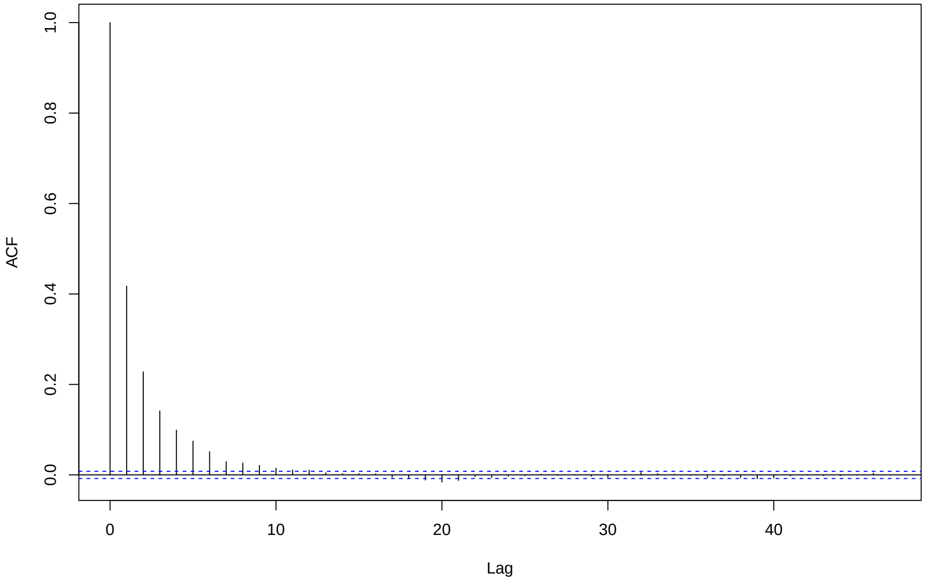
ACF for eta[5,5]
