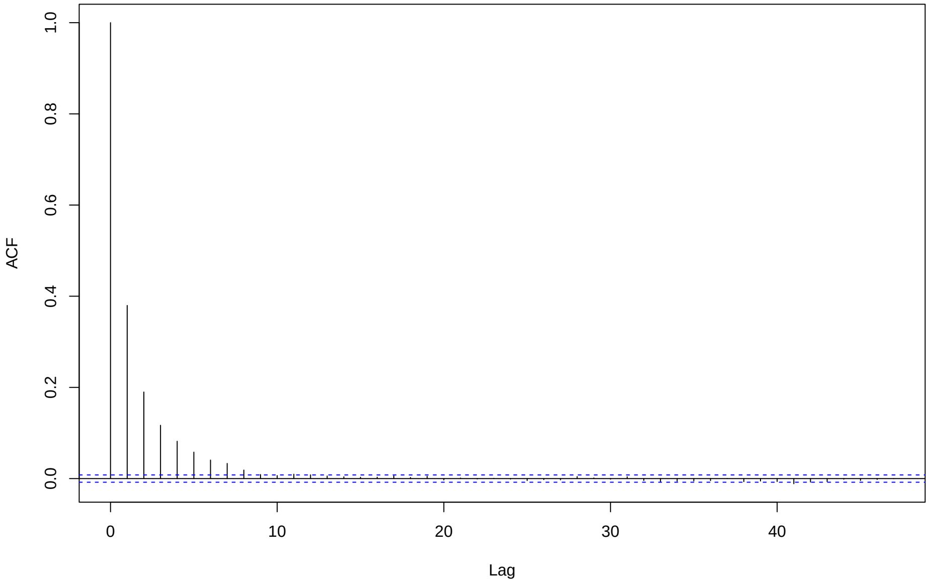
ACF for eta[5,2]
