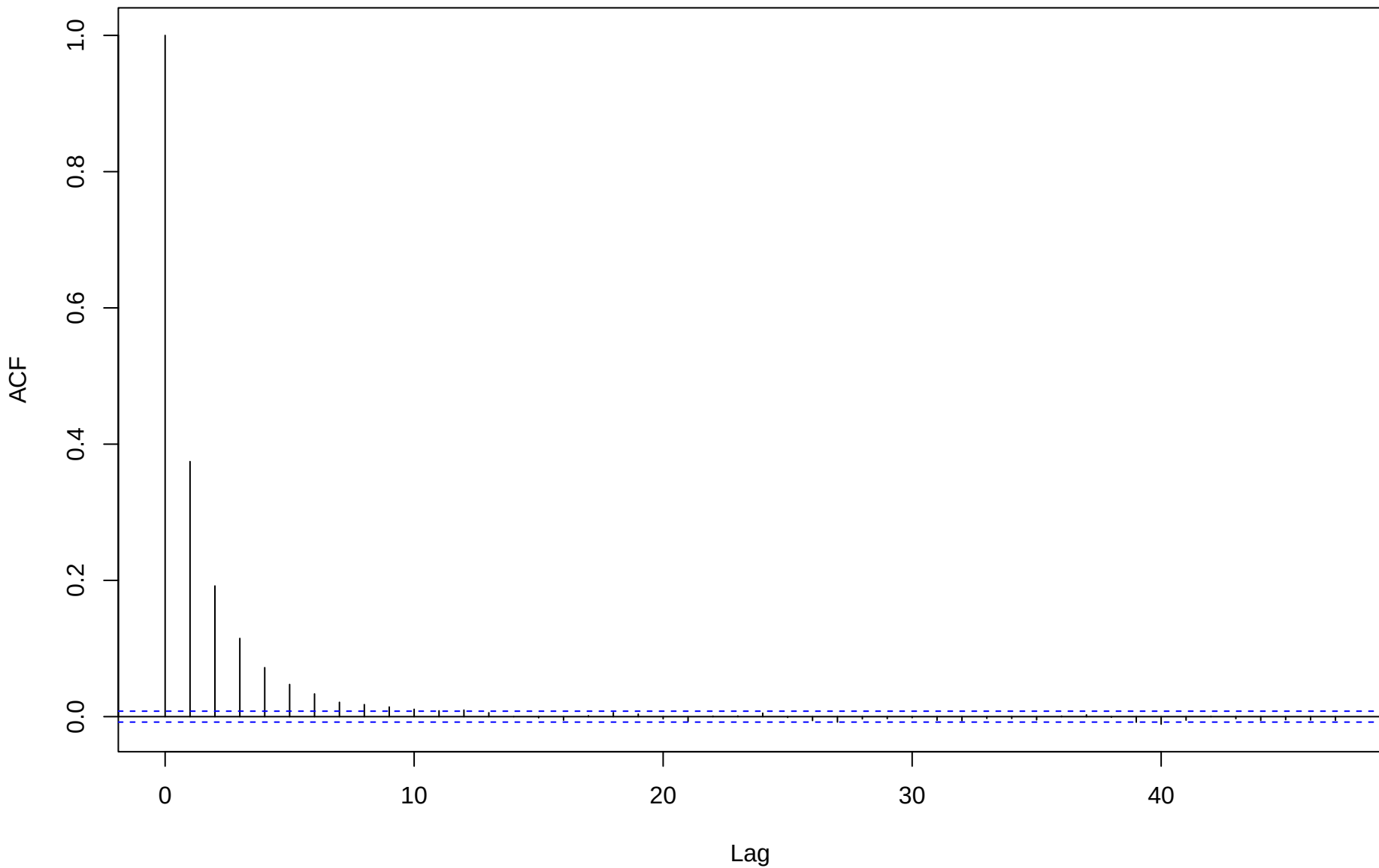
ACF for eta[3,4]
