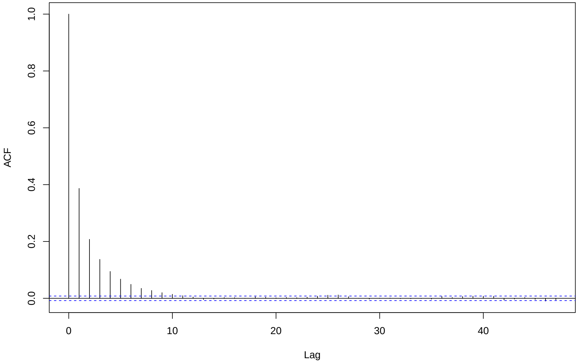
ACF for eta[1,7]
