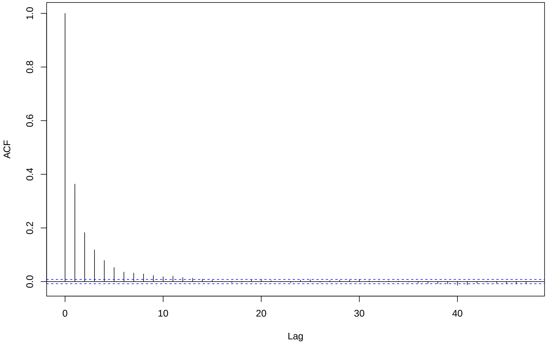
ACF for eta[2,5]
