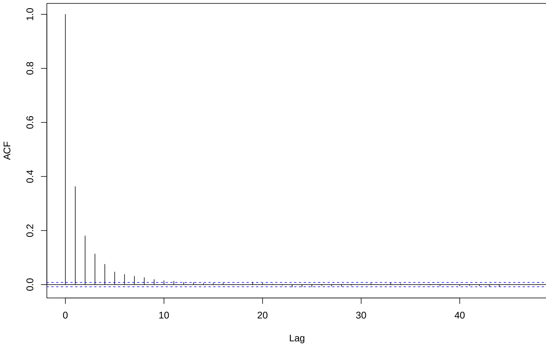
ACF for eta[5,10]
