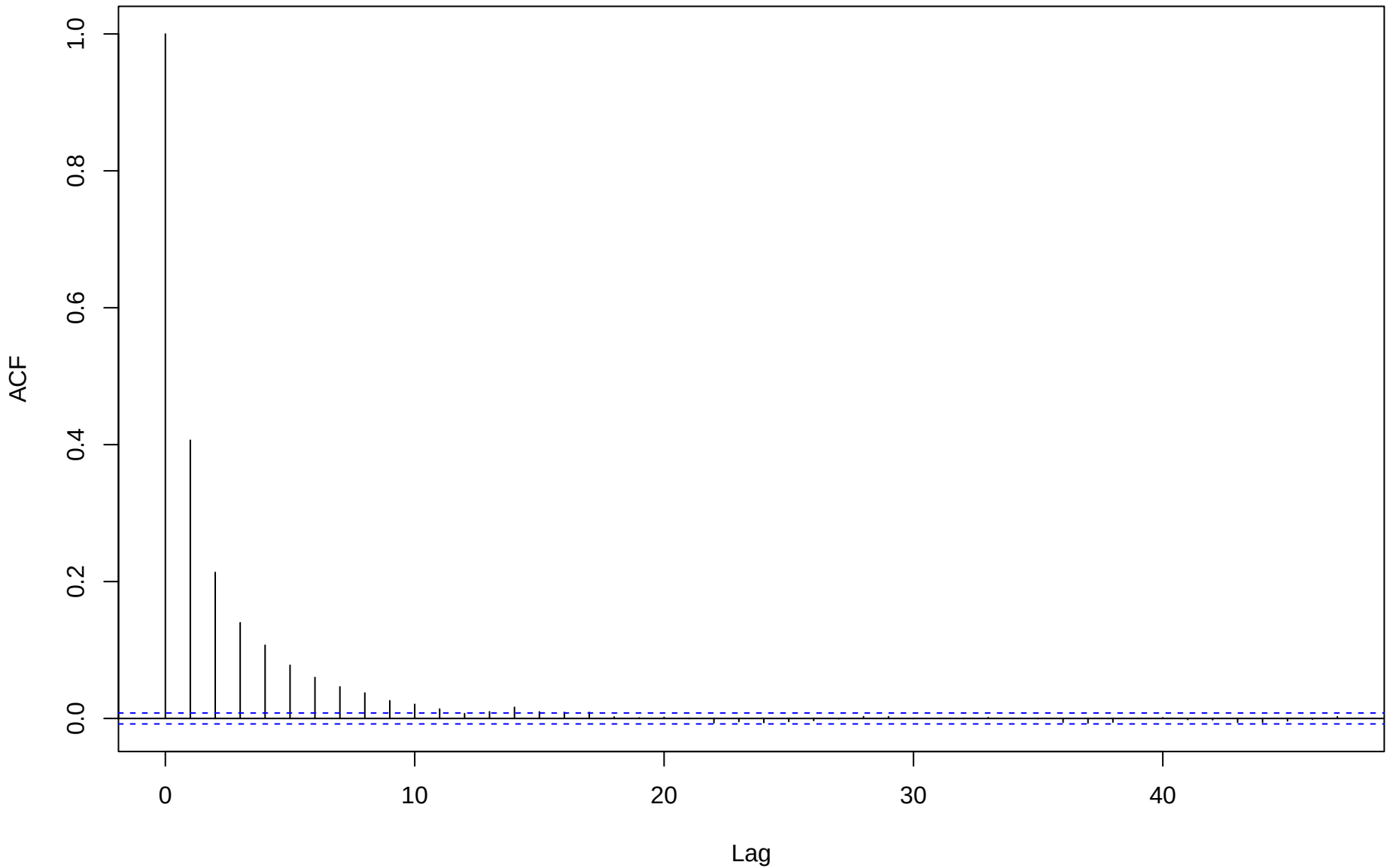
ACF for eta[4,3]
