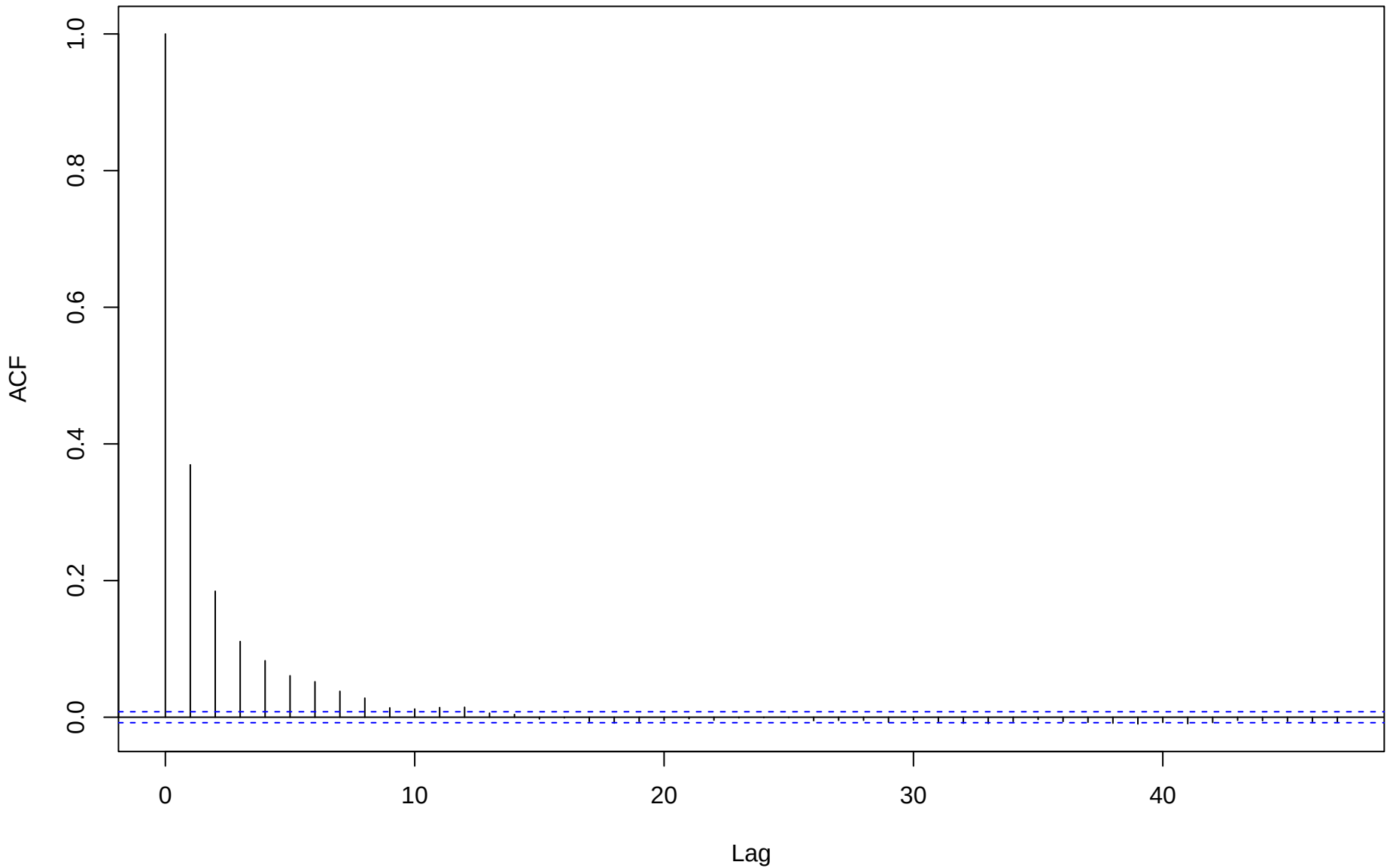
ACF for eta[2,4]
