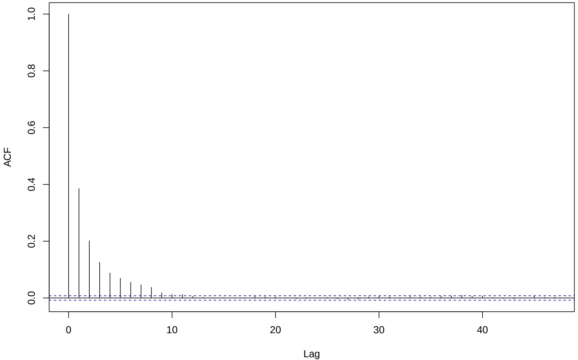
ACF for eta[1,3]
