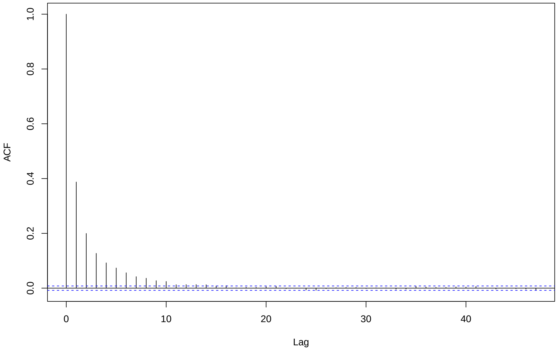
ACF for eta[4,5]
