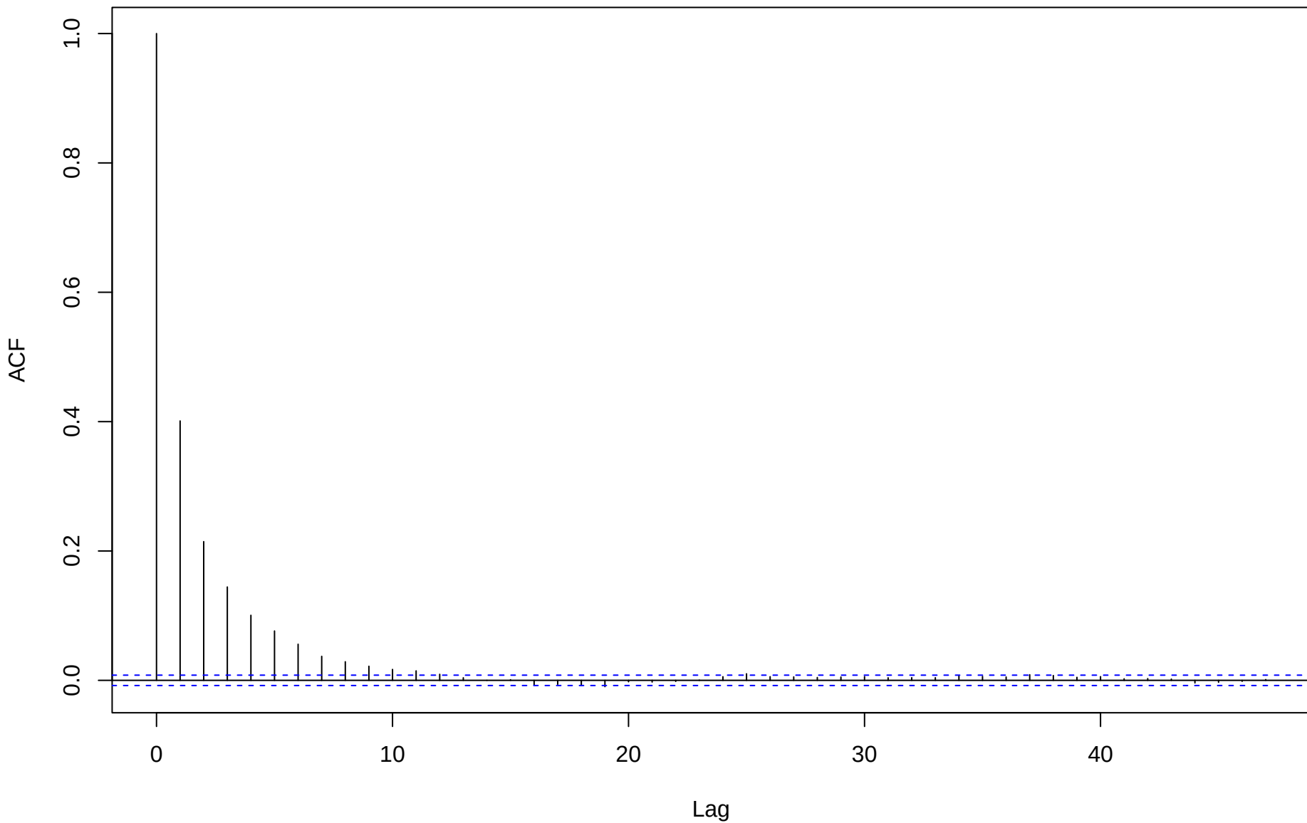
ACF for eta[1,1]
