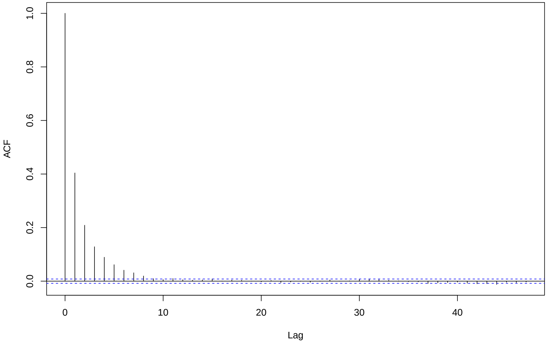
ACF for eta[3,5]
