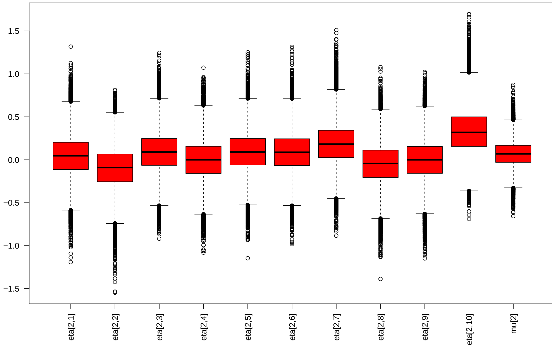
Posterior Boxplots for Sector 2 and mu
