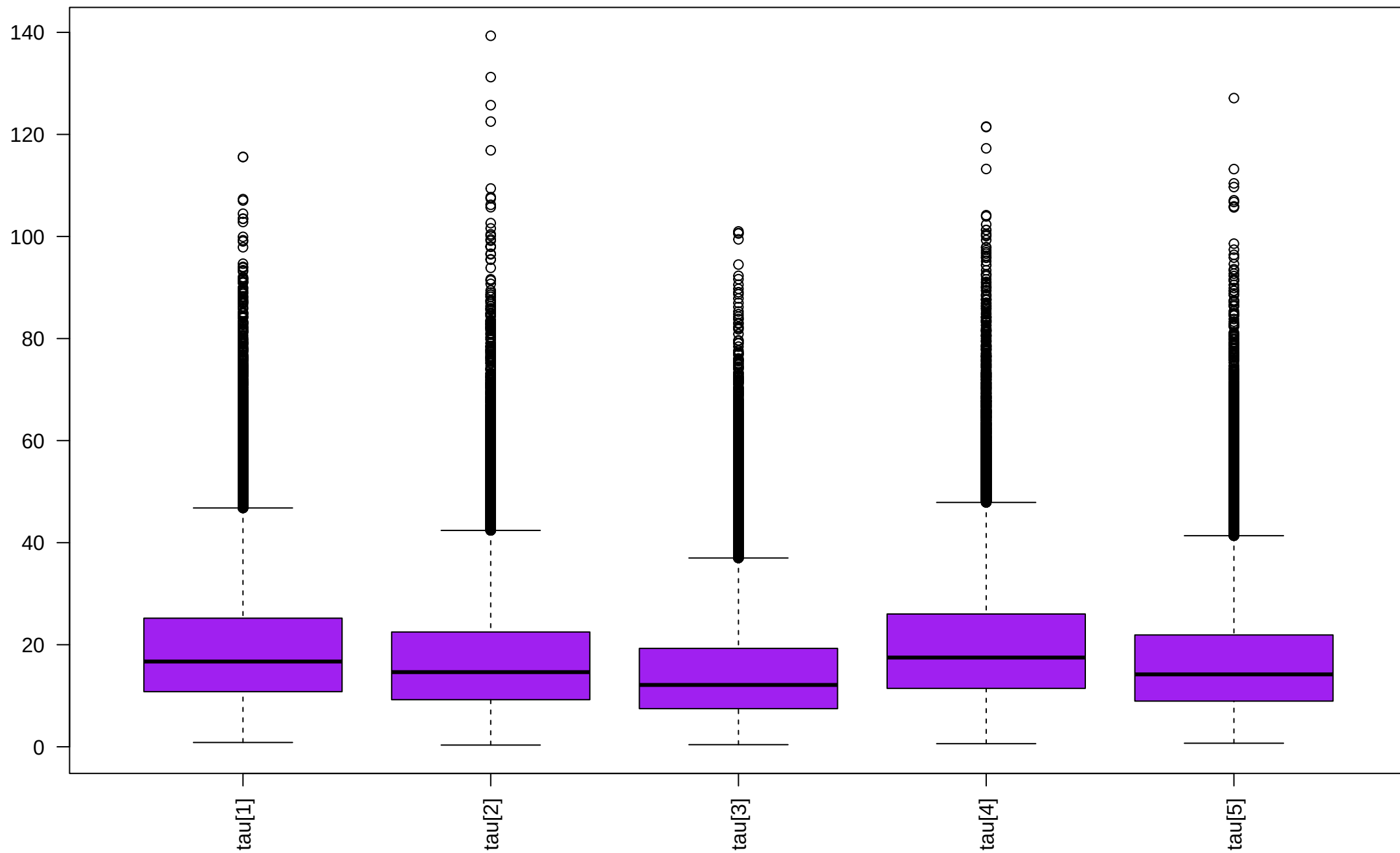
Posterior Boxplots for tau
