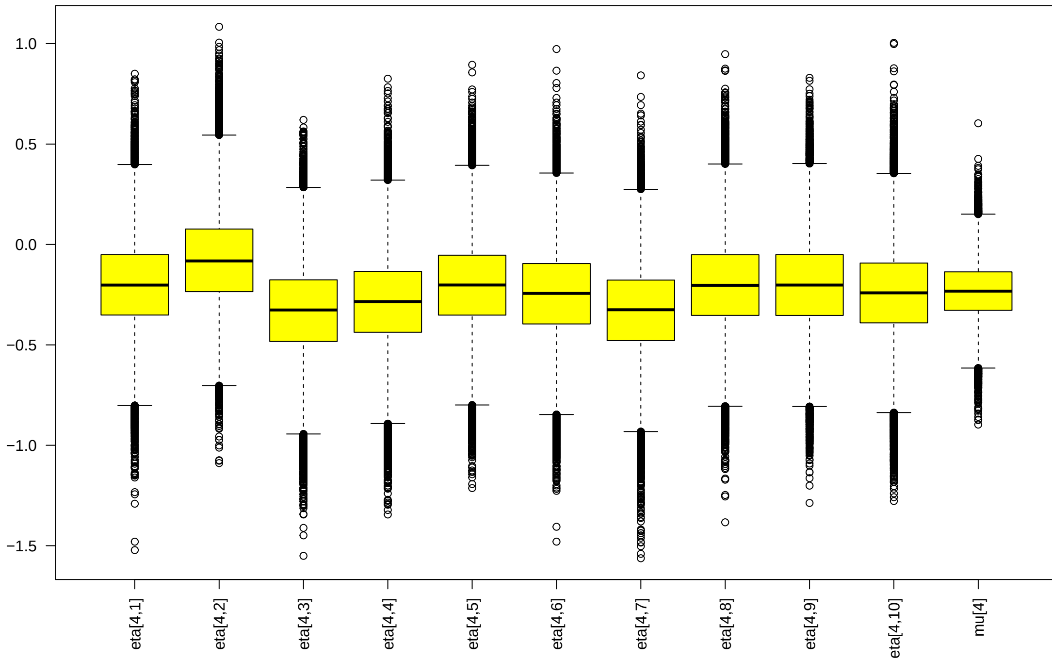
Posterior Boxplots for Sector 4 and mu
