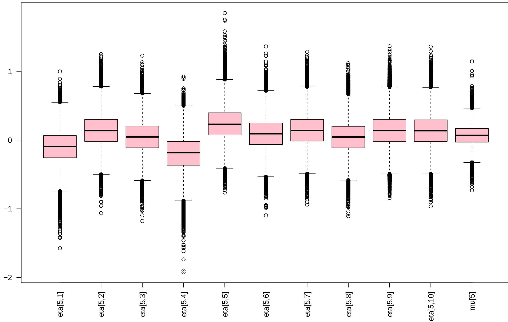
Posterior Boxplots for Sector 5 and mu
