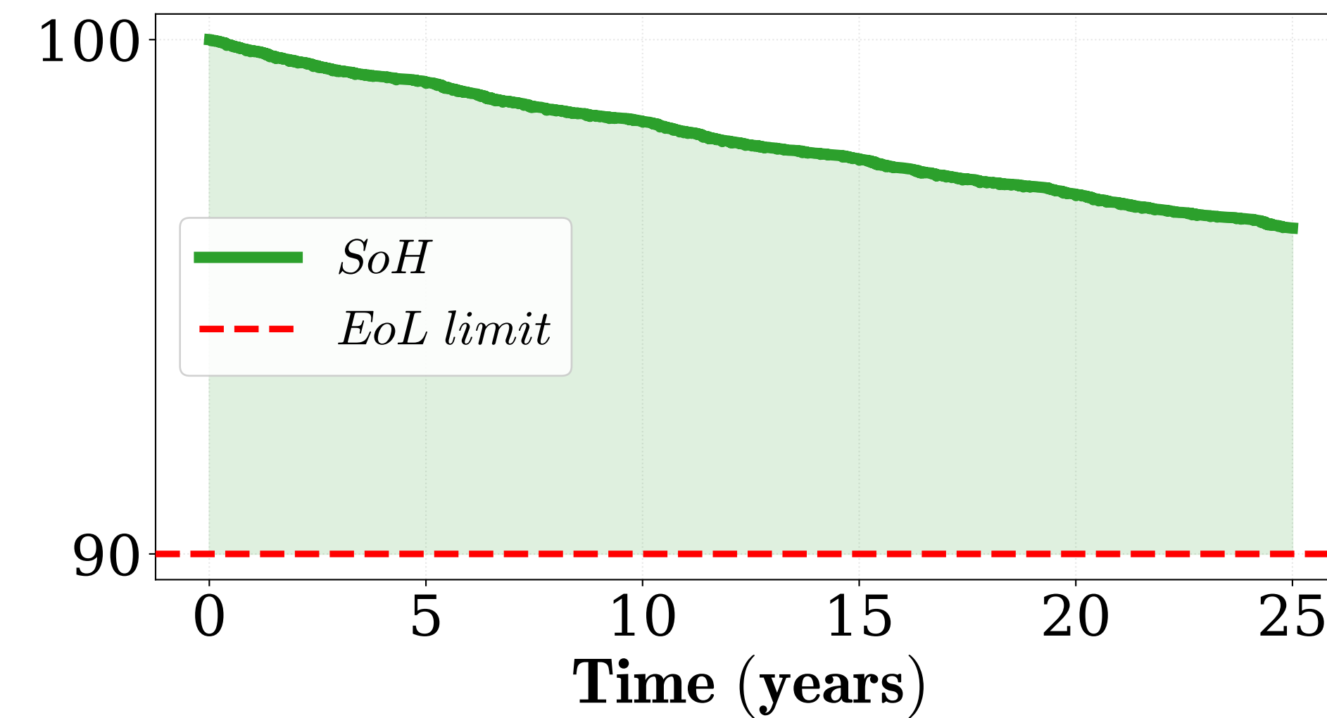
PEMWE Degradation
