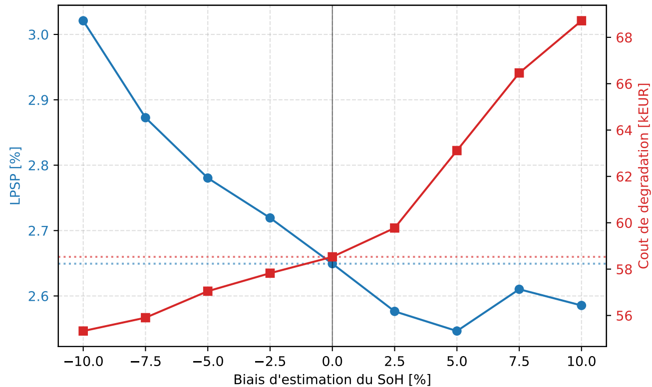
Biais d'estimation du SoH
