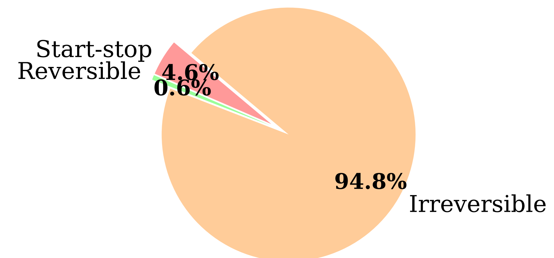
PEMWE Degradation
