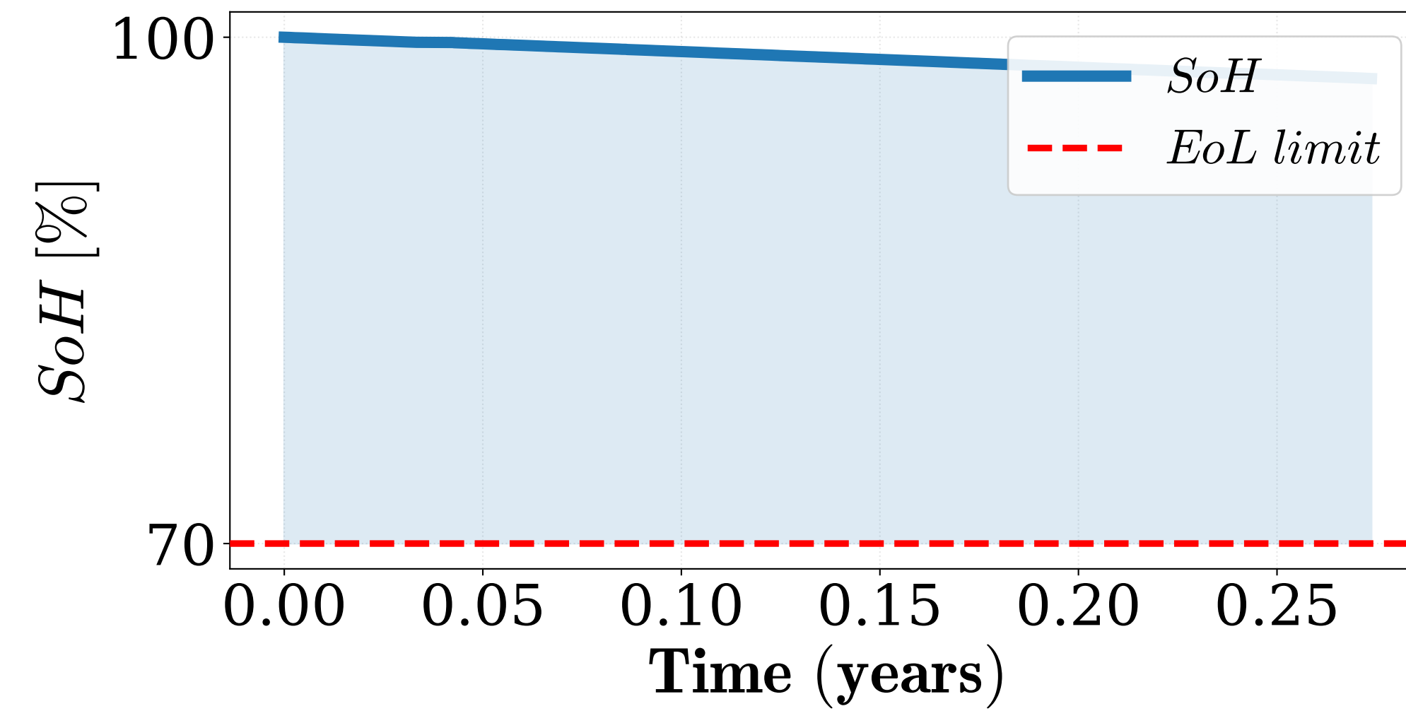
PEMFC Degradation
