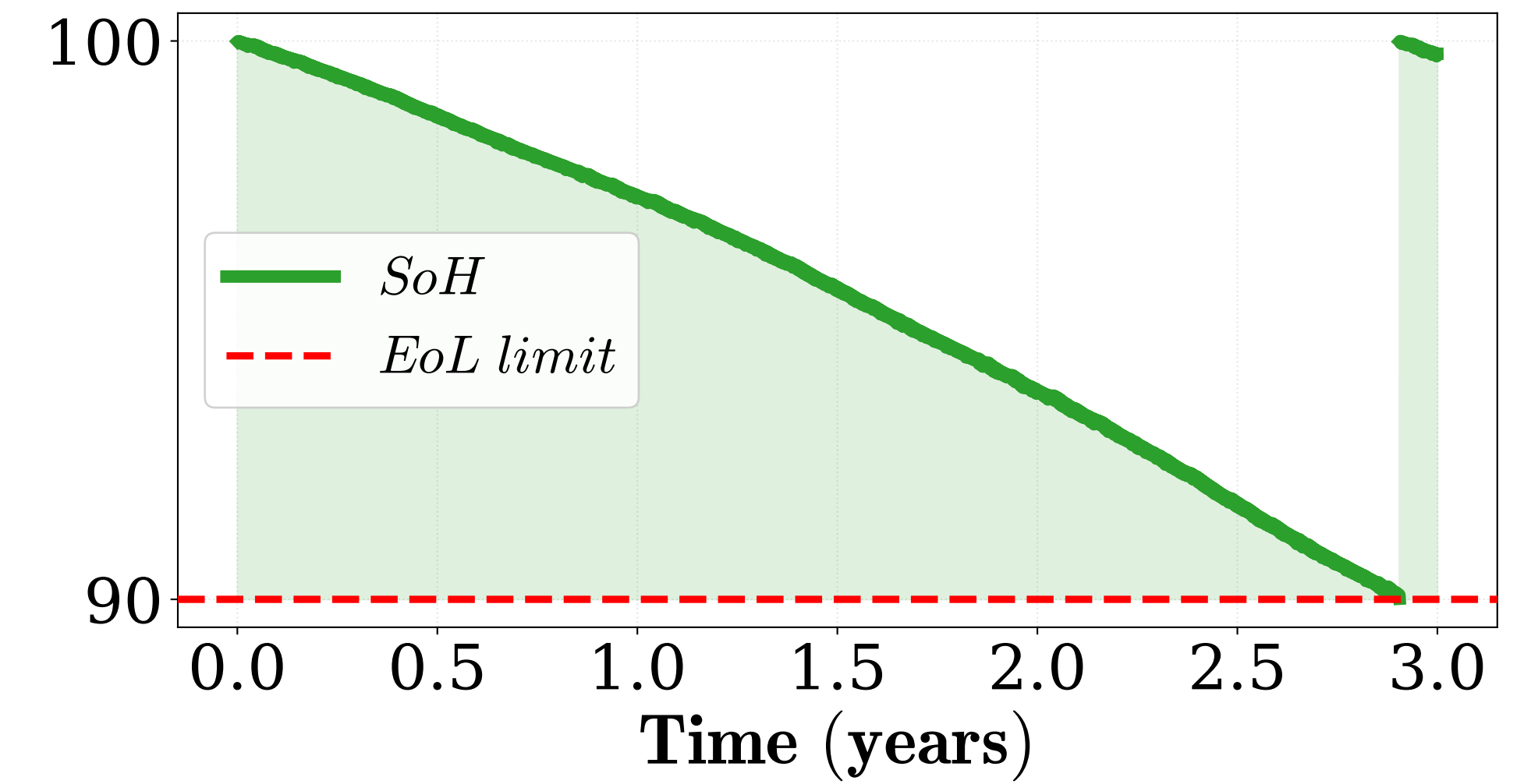
PEMWE Degradation
