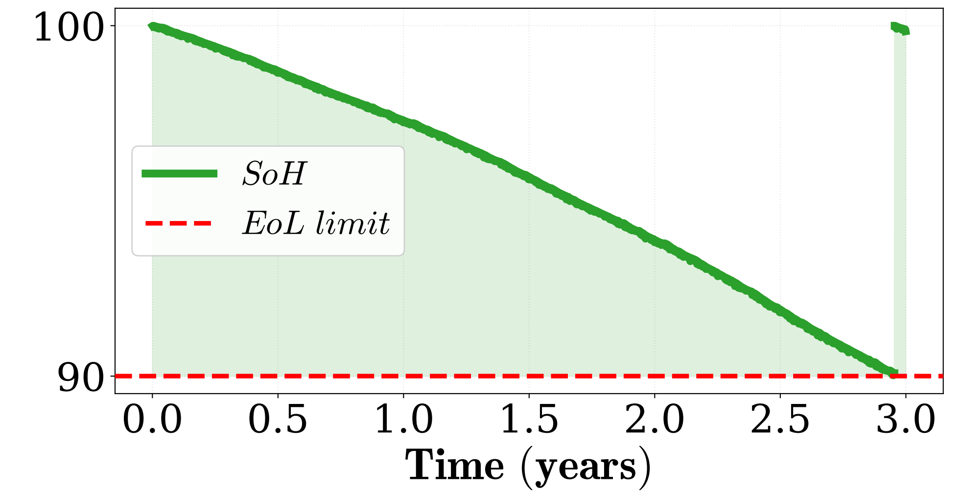
PEMWE Degradation
