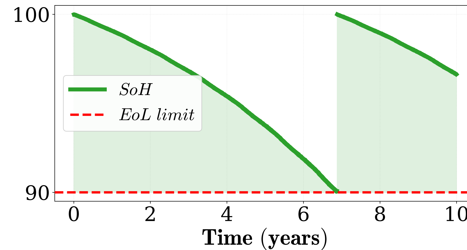
PEMWE Degradation
