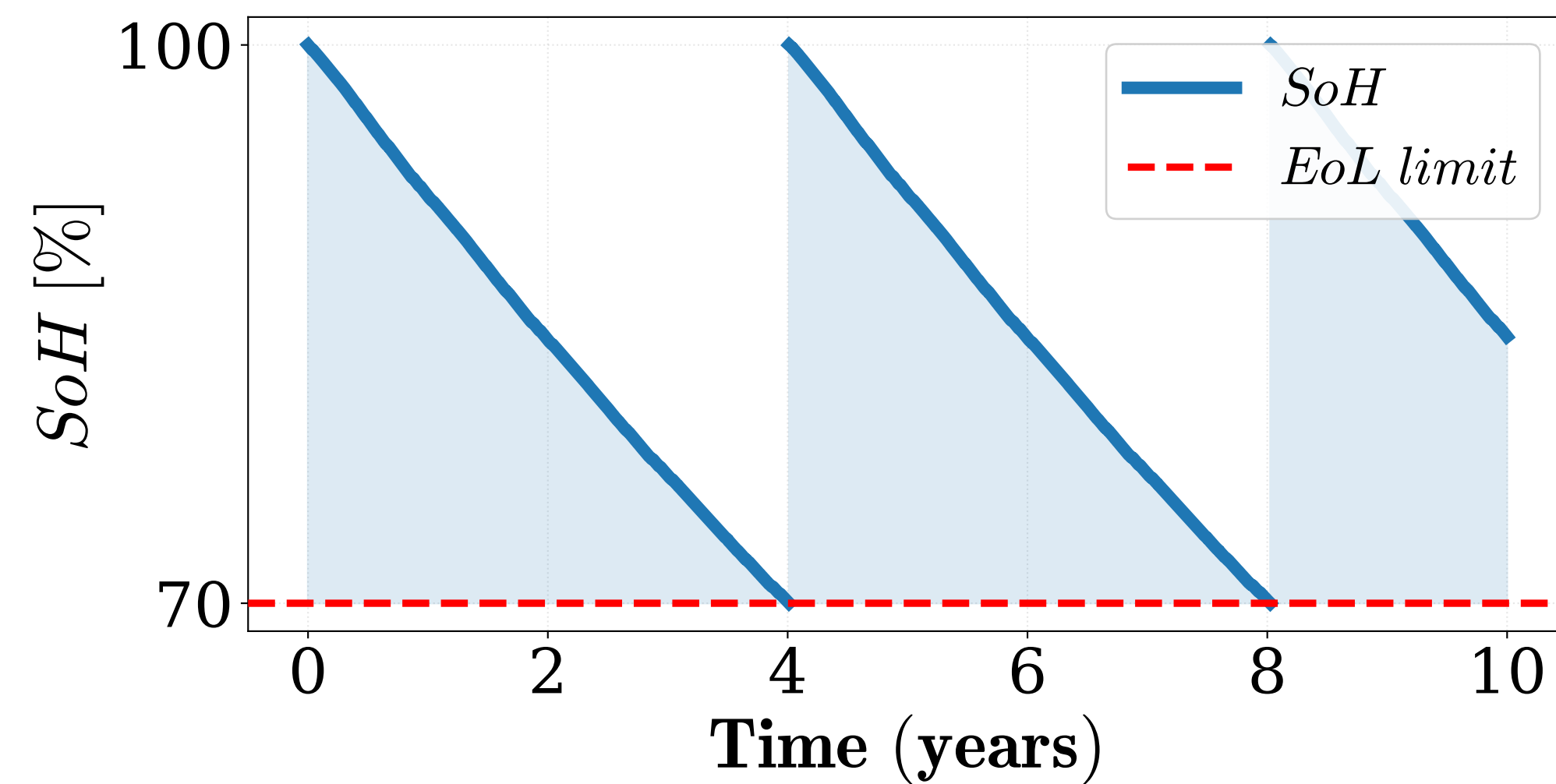
PEMFC Degradation
