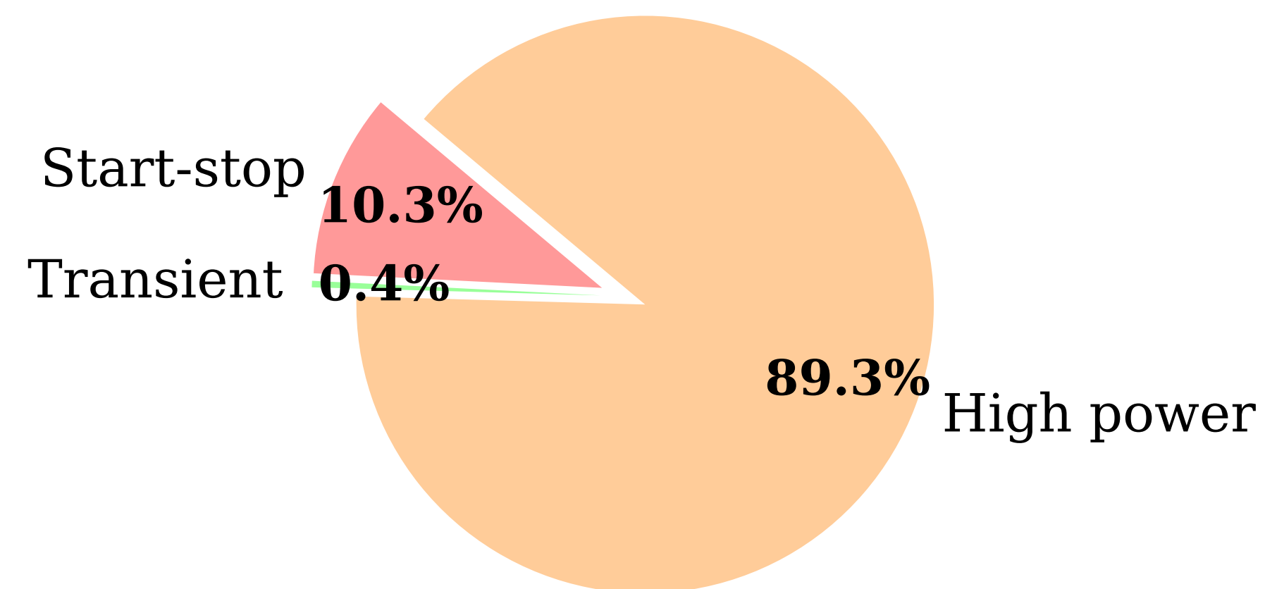
PEMFC Degradation
