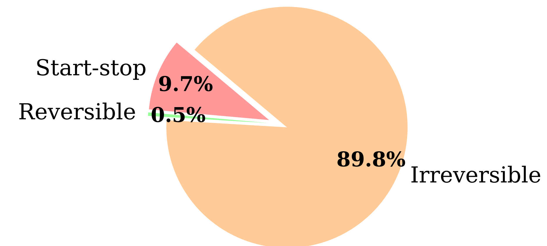
PEMWE Degradation
