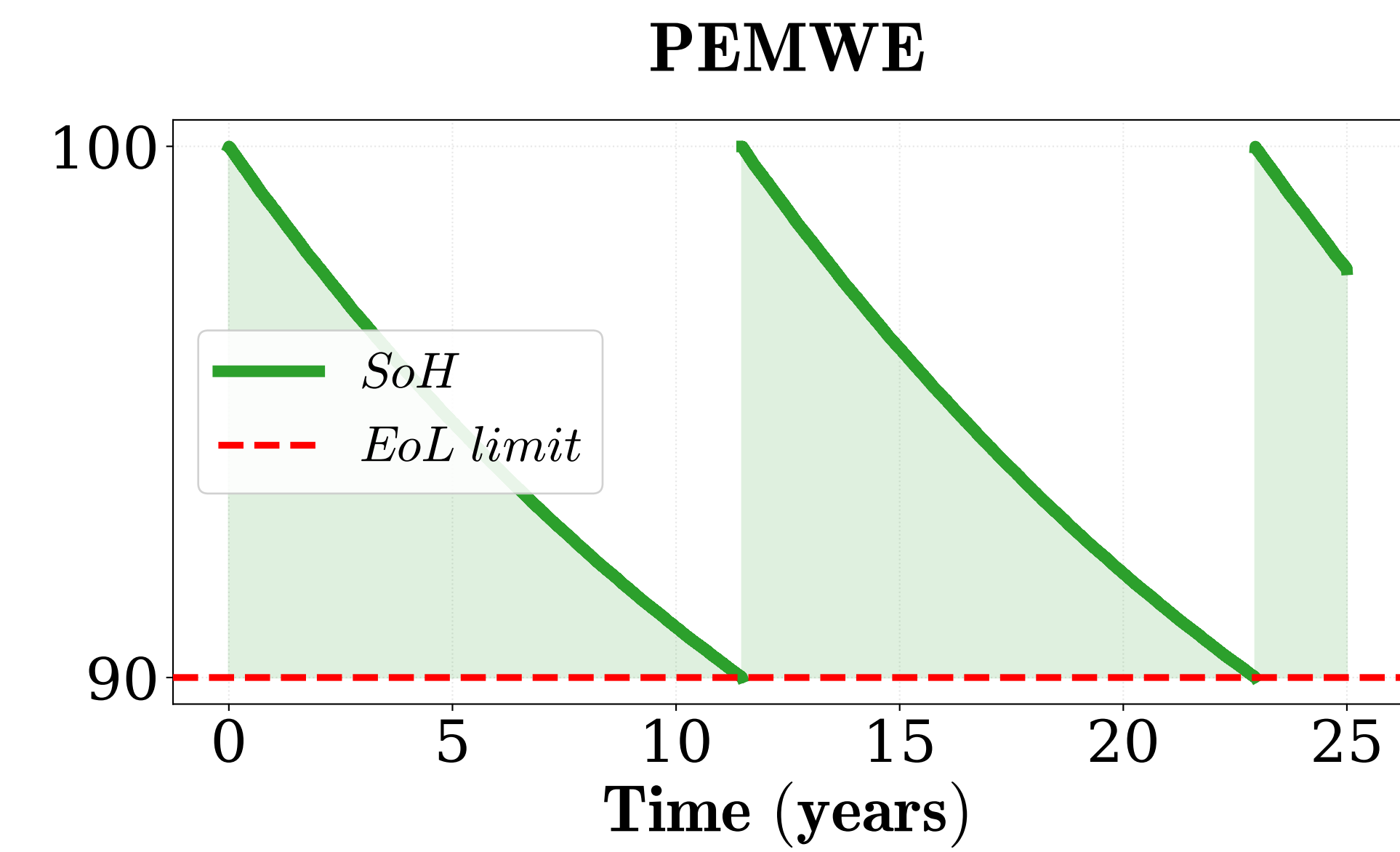
PEMWE Degradation
