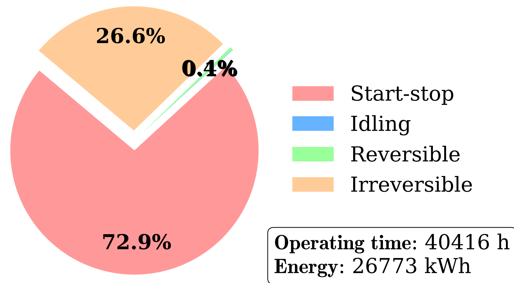
PEMFC Degradation
