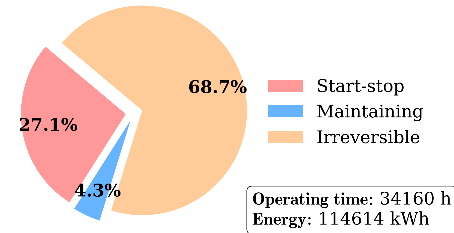
PEMWE Degradation
