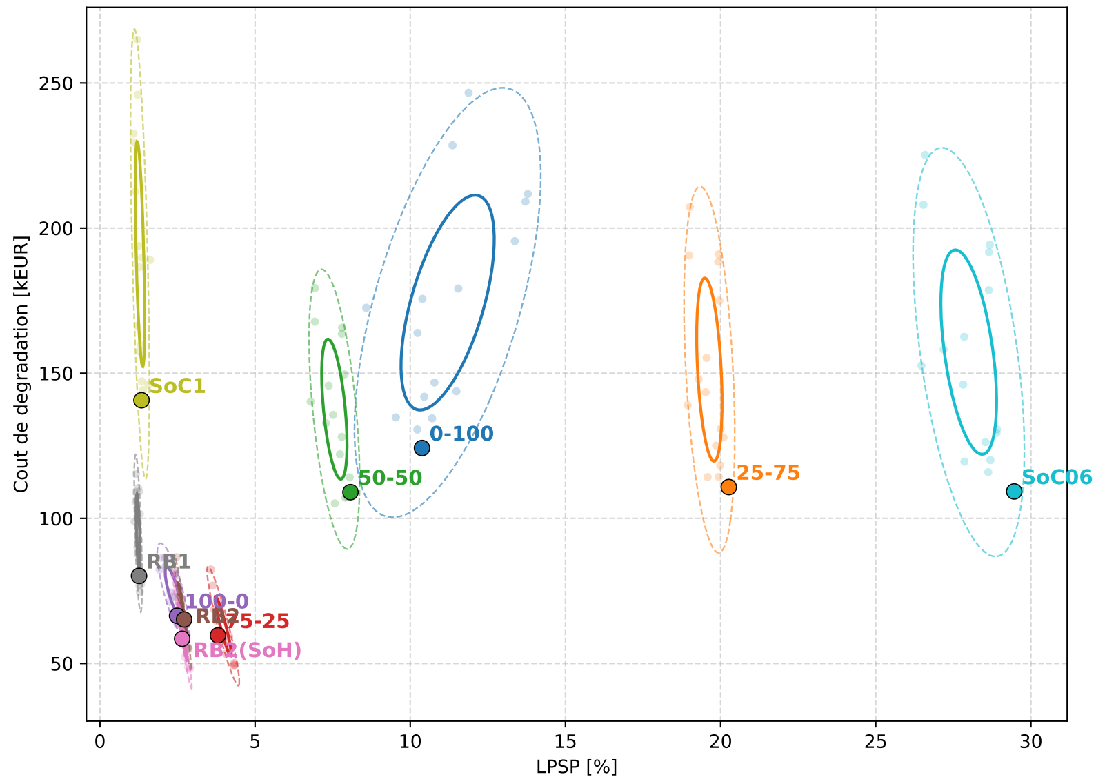
Robustesse du front de Pareto aux seuils de fin de vie (EoL) point = seuils nominaux ; ellipses 1\sigma/2\sigma = incertitude EoL (bat 0.60-0.80, FC/ELY 0.90-0.96)
