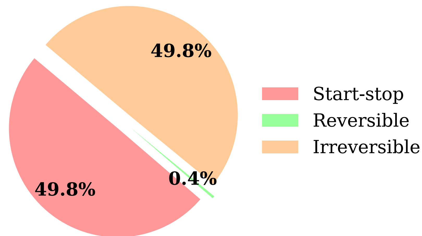
PEMFC Degradation
