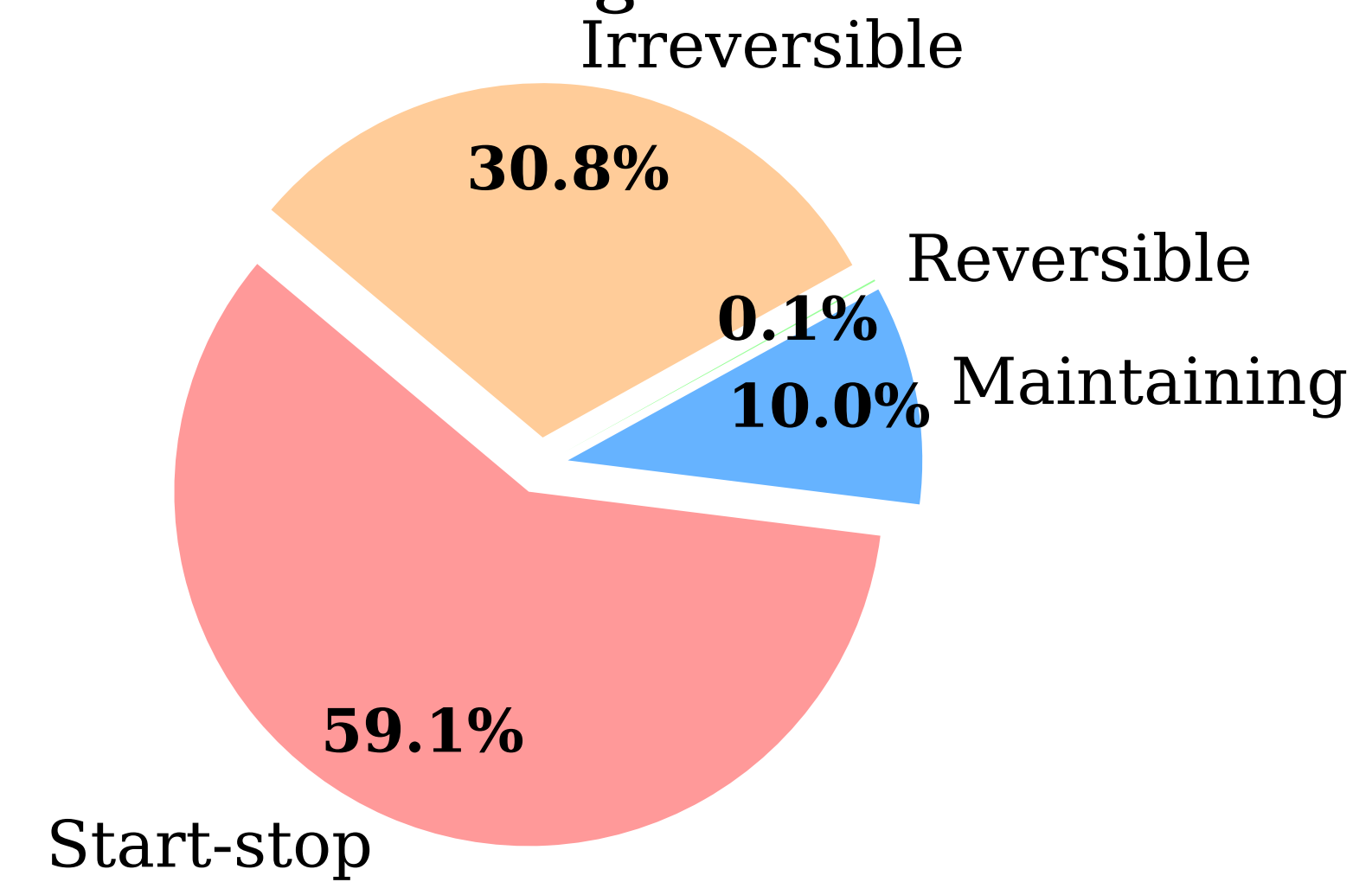
PEMWE Degradation
