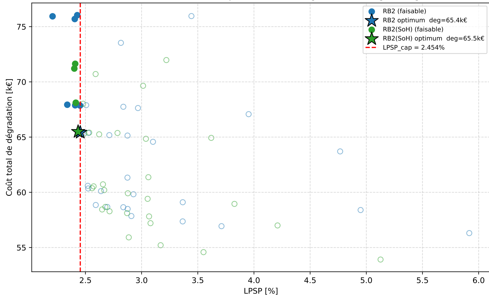
RB2 vs RB2(SoH) — min dégradation sous contrainte LPSP (25 ans) même moteur, même métrique ; faisable = à gauche de la ligne rouge
