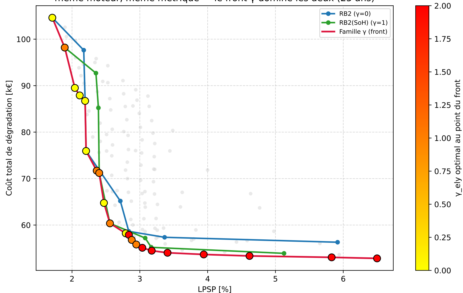
Famille \gamma ( P=c \cdot P_{\max} \cdot \text{SoH}^\gamma ) niche RB2 ( \gamma=0 ) et RB2(SoH) ( \gamma=1 ) même moteur, même métrique — le front \gamma domine les deux (25 ans)
