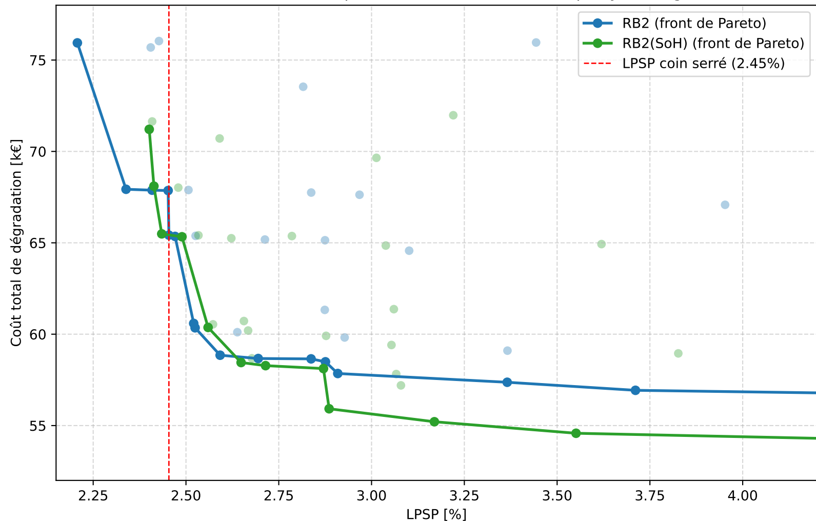
RB2 vs RB2(SoH) — fronts de Pareto LPSP-dégradation (25 ans) même moteur, même métrique ; RB2(SoH) domine dès qu'il y a marge de LPSP
