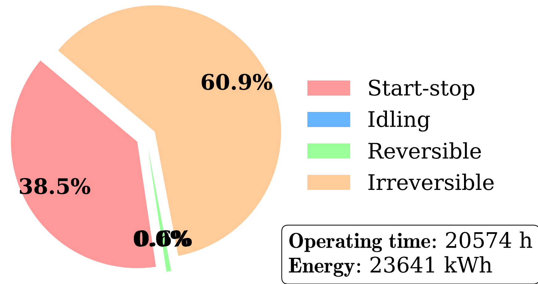
PEMFC Degradation
