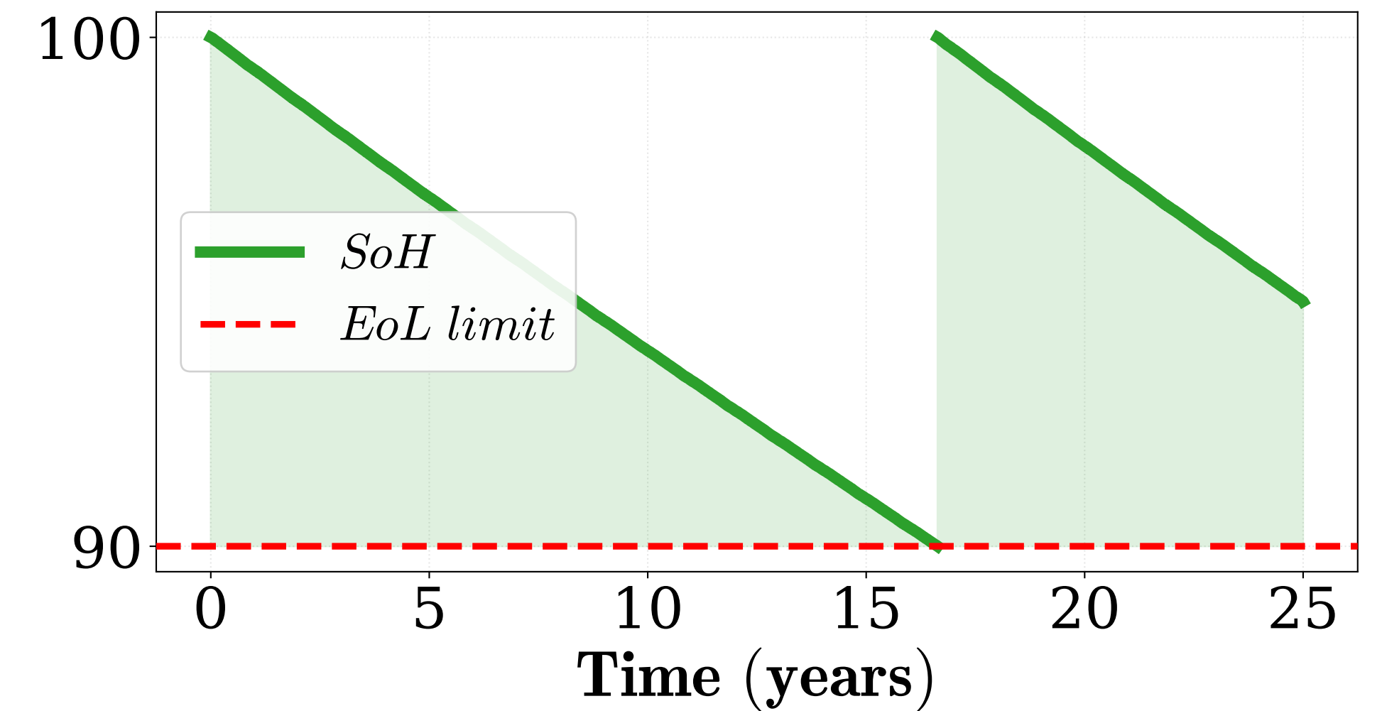
PEMWE Degradation
