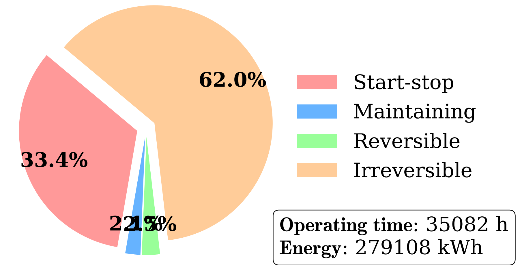
PEMWE Degradation
