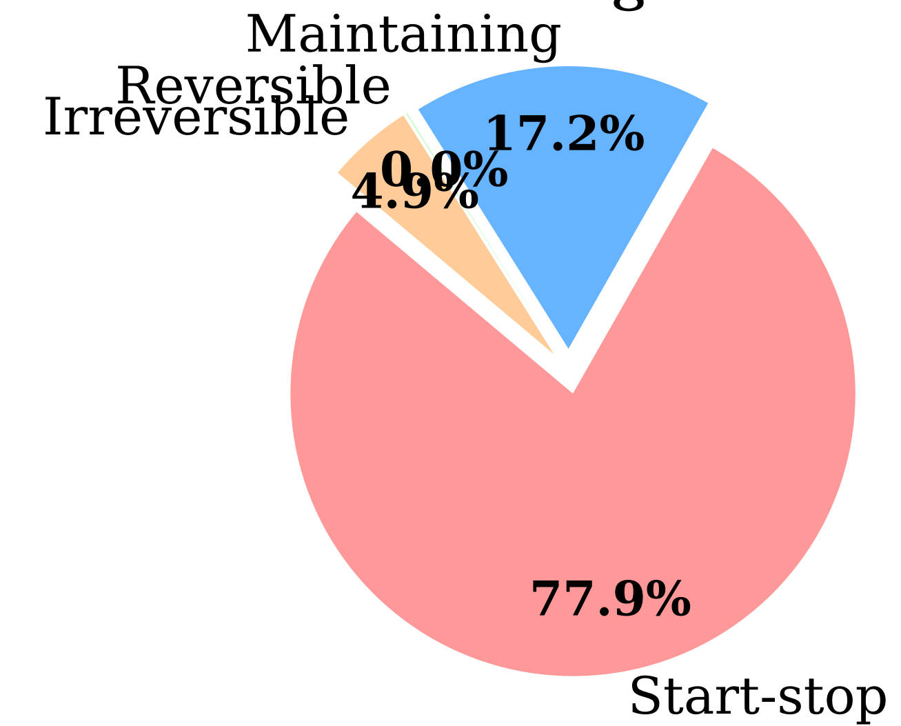
PEMWE Degradation
