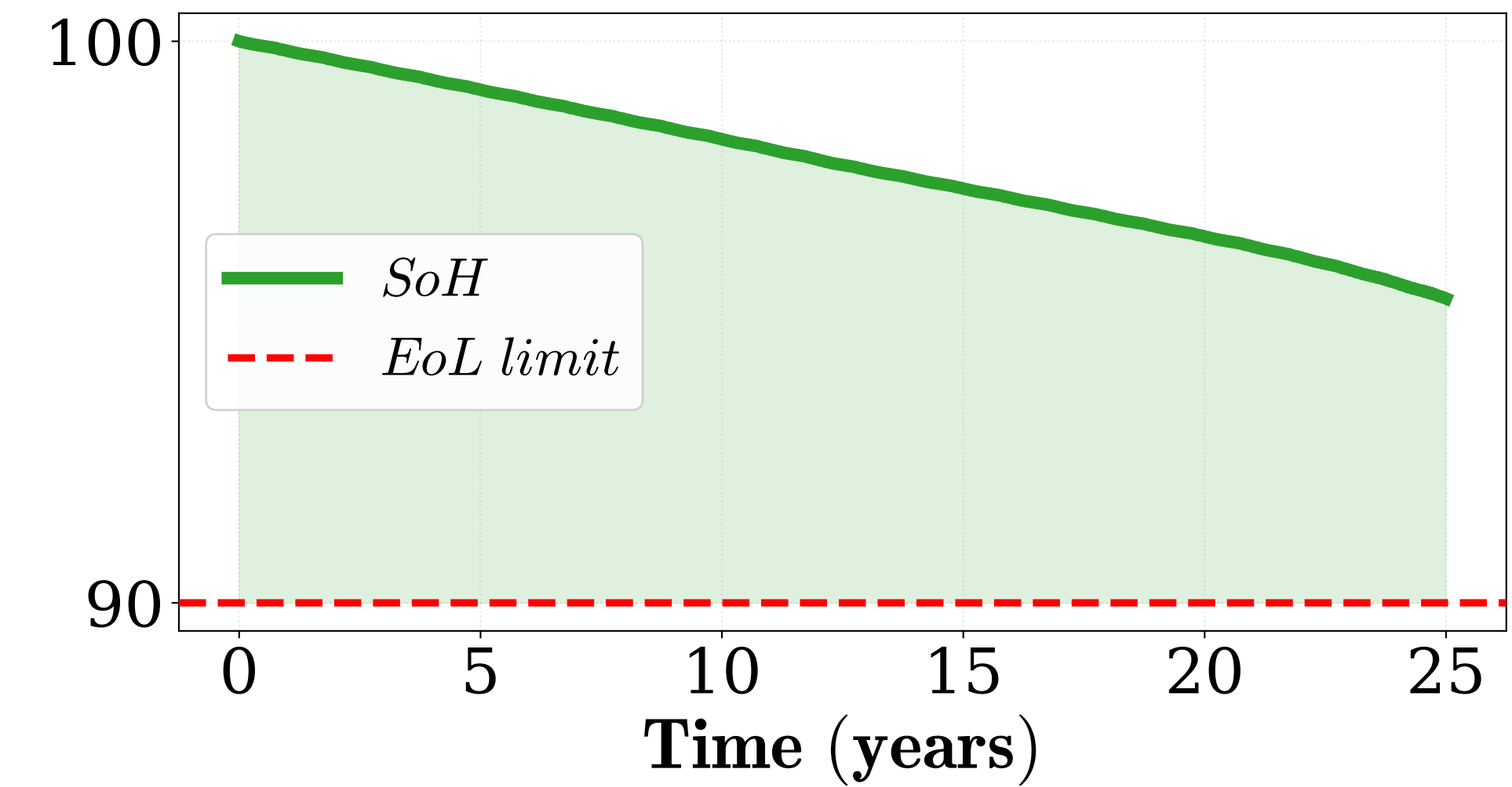
PEMWE Degradation
