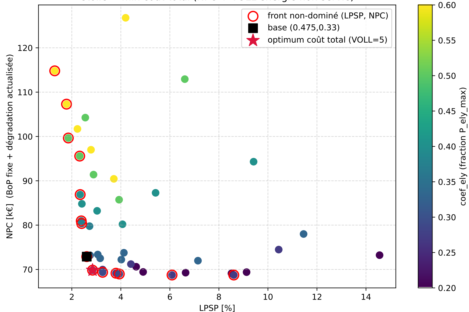
RB2(SoH) — setpoints à dimensionnement fixé (25 ans) étoile = min coût total (NPC + VOLL·énergie non servie)
