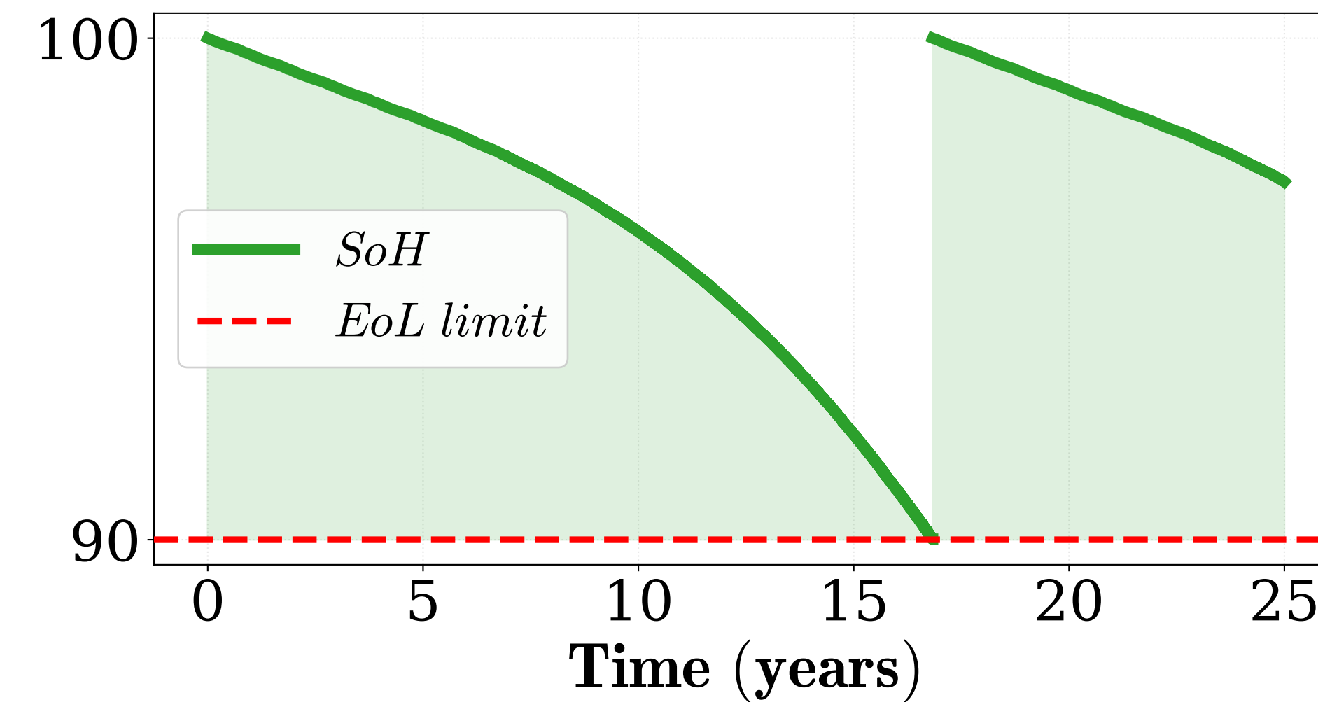
PEMWE Degradation
