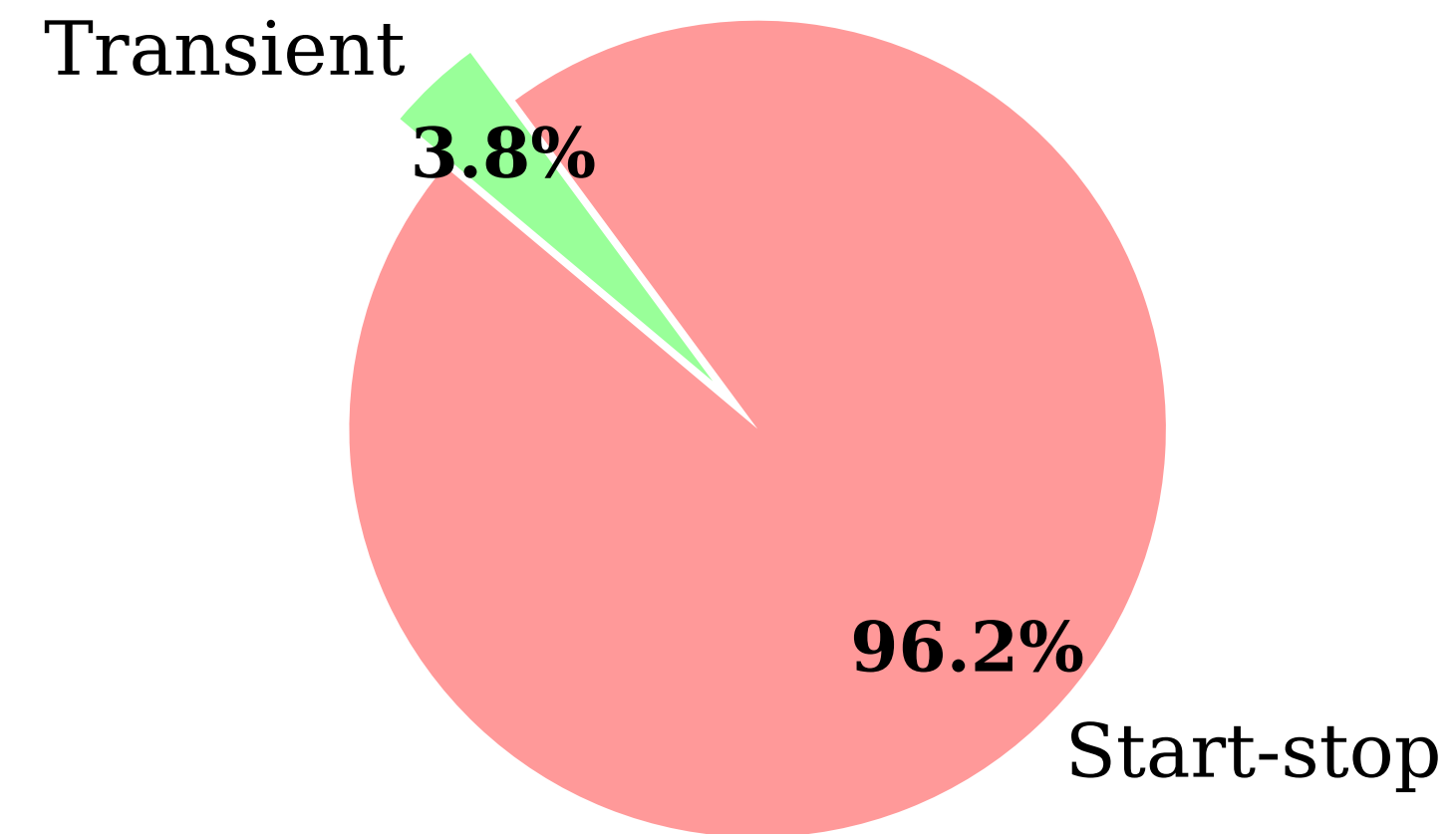
PEMFC Degradation
