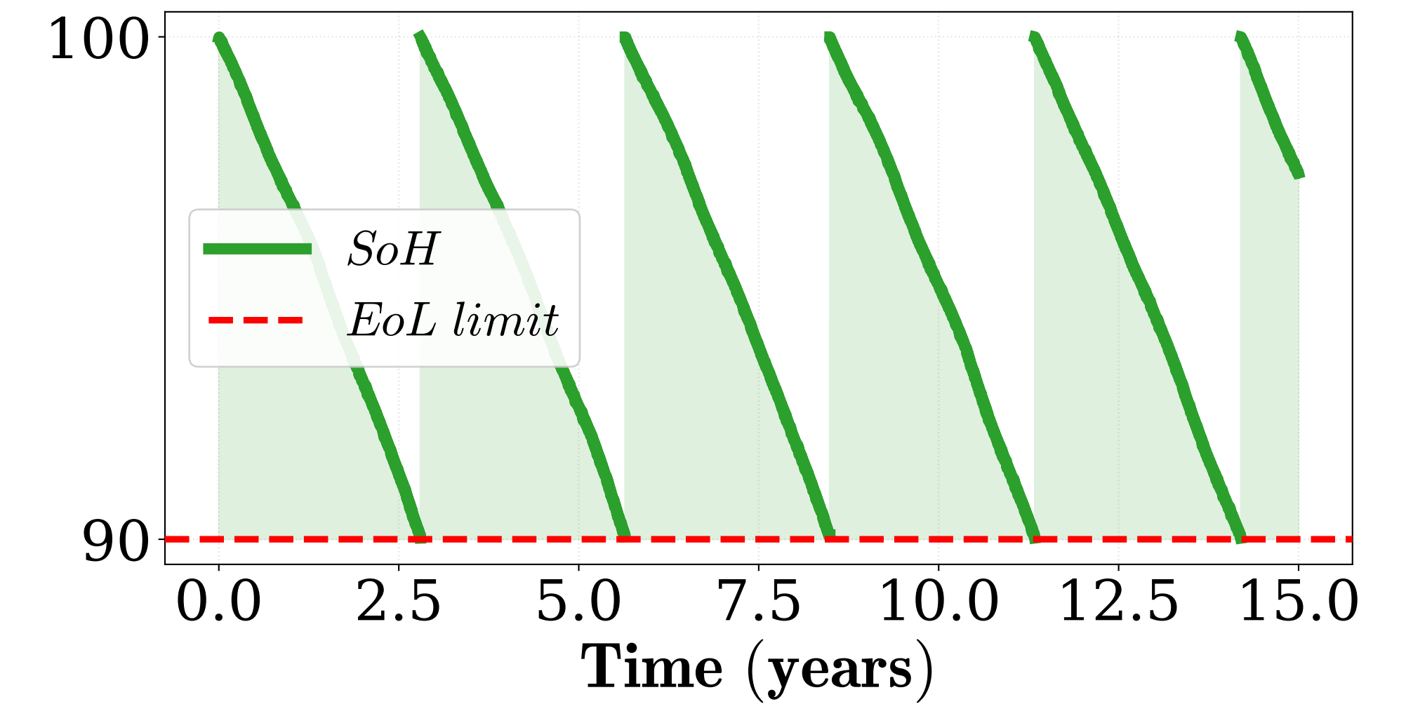
PEMWE Degradation
