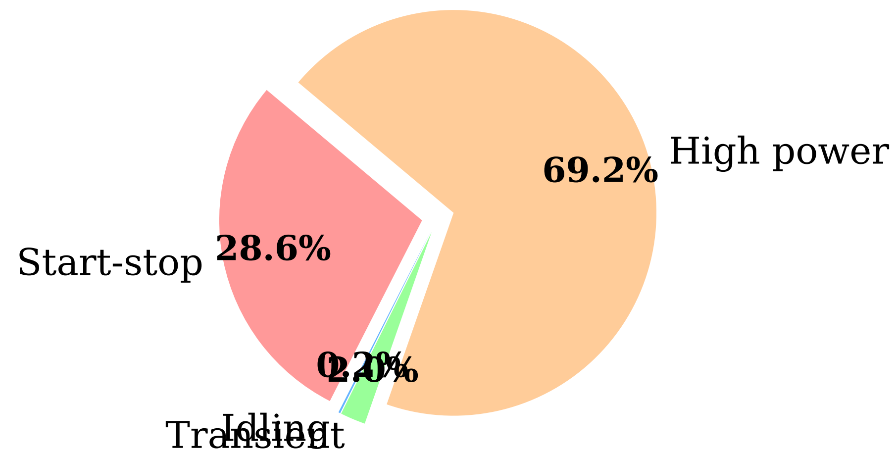
PEMFC Degradation
