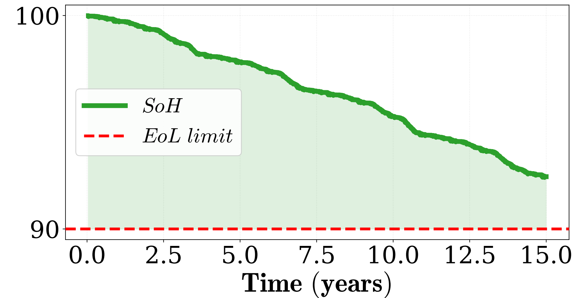
PEMWE Degradation
