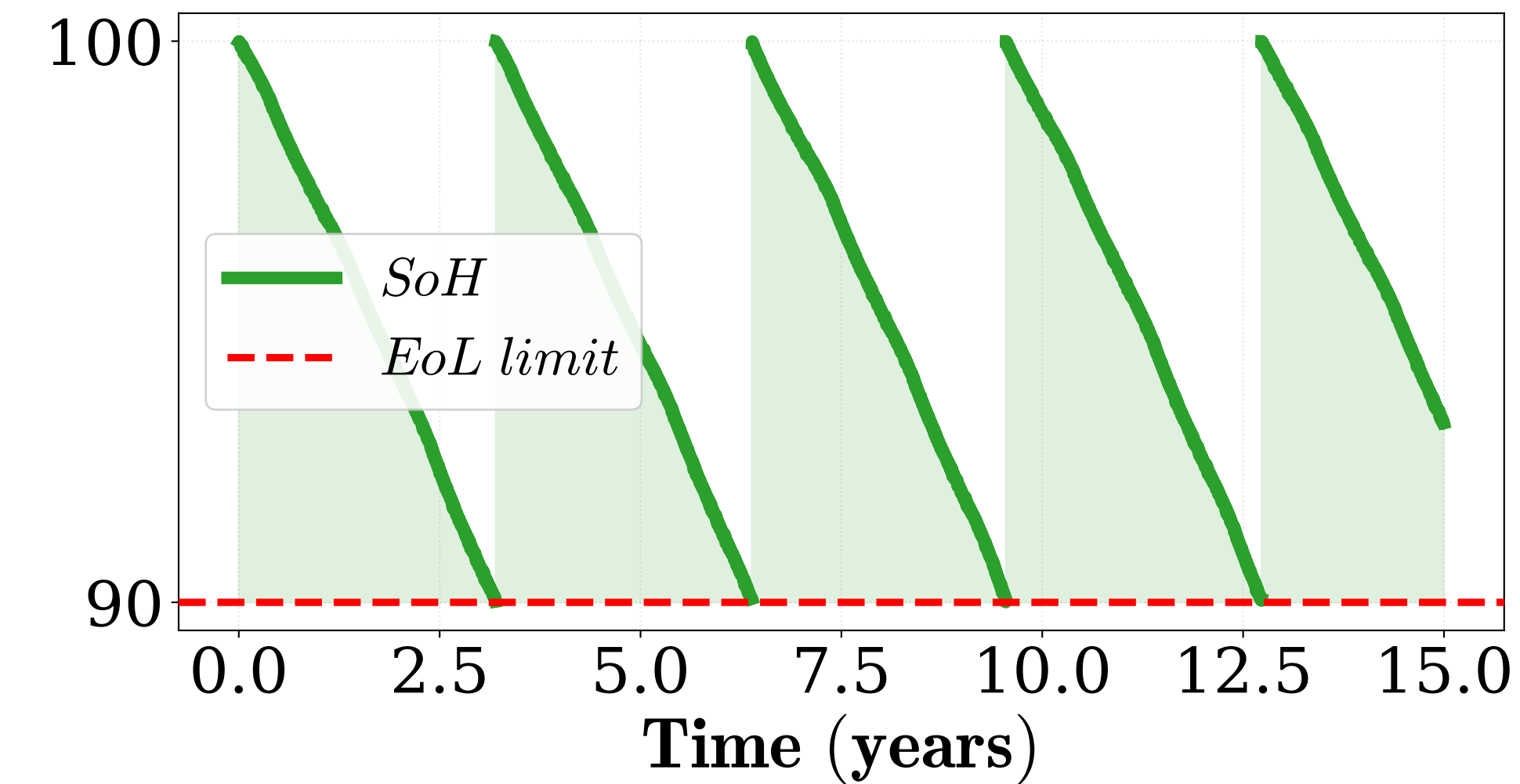
PEMWE Degradation
