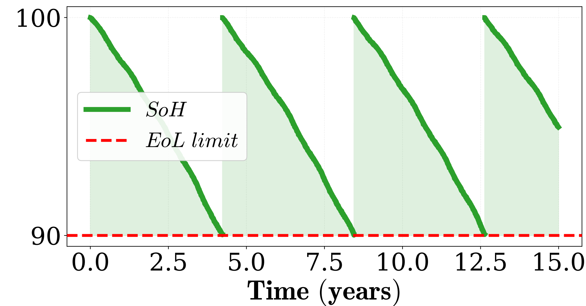
PEMWE Degradation
