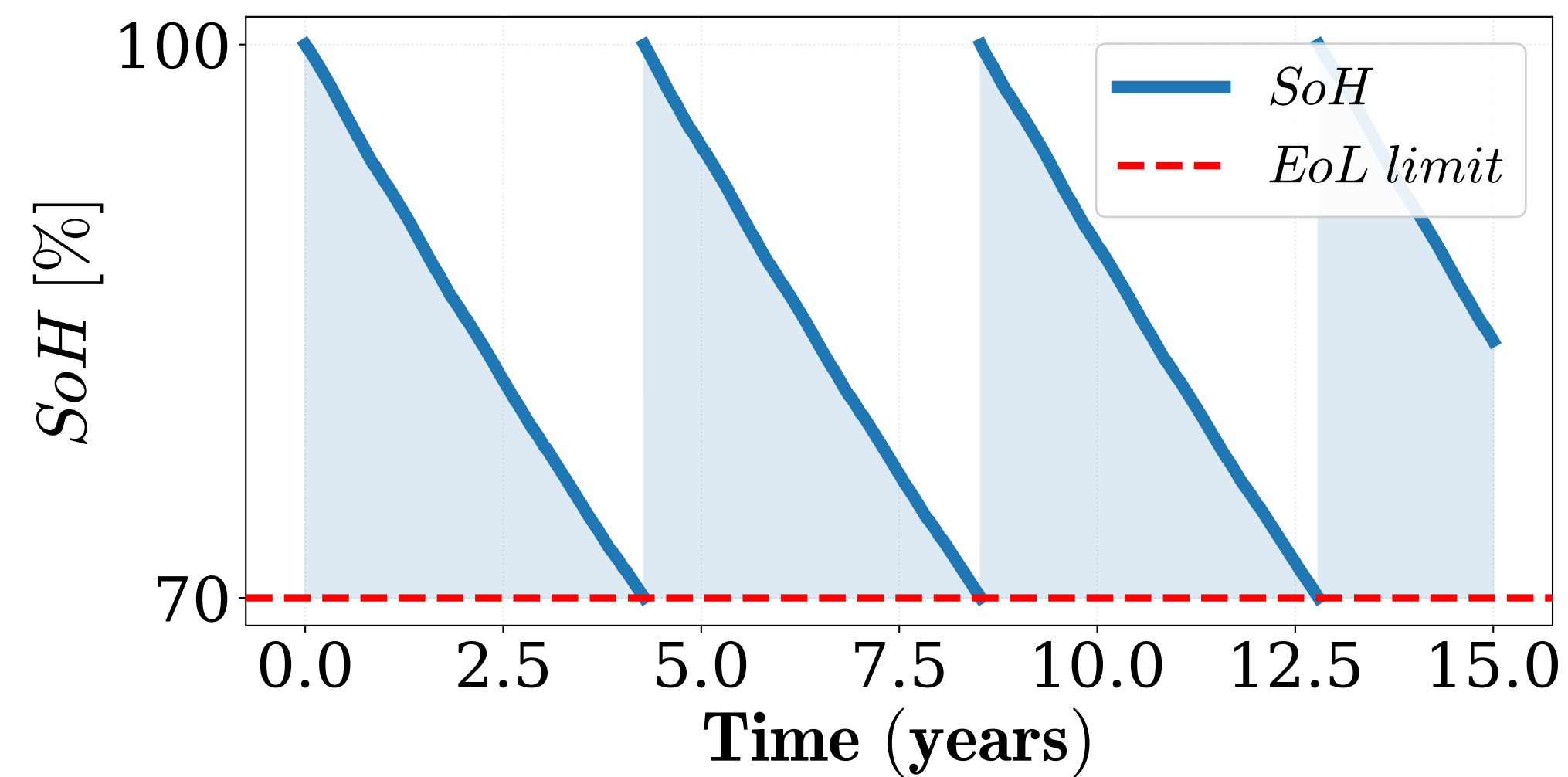
PEMFC Degradation
