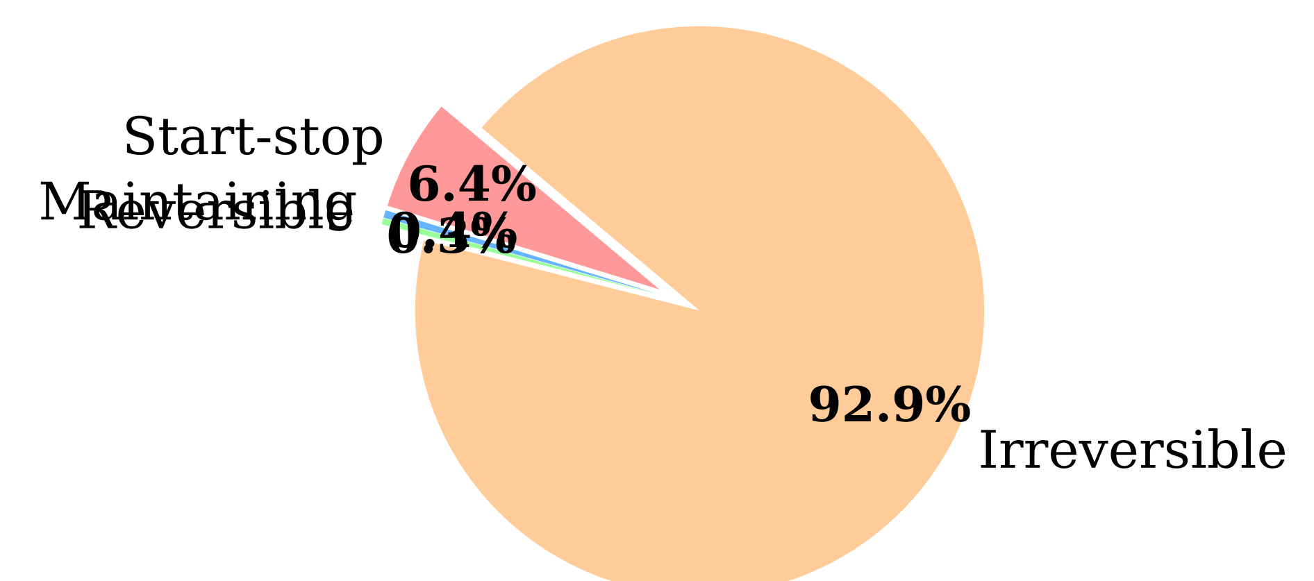
PEMWE Degradation
