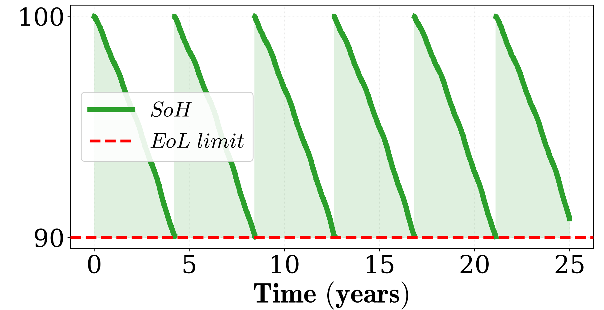
PEMWE Degradation
