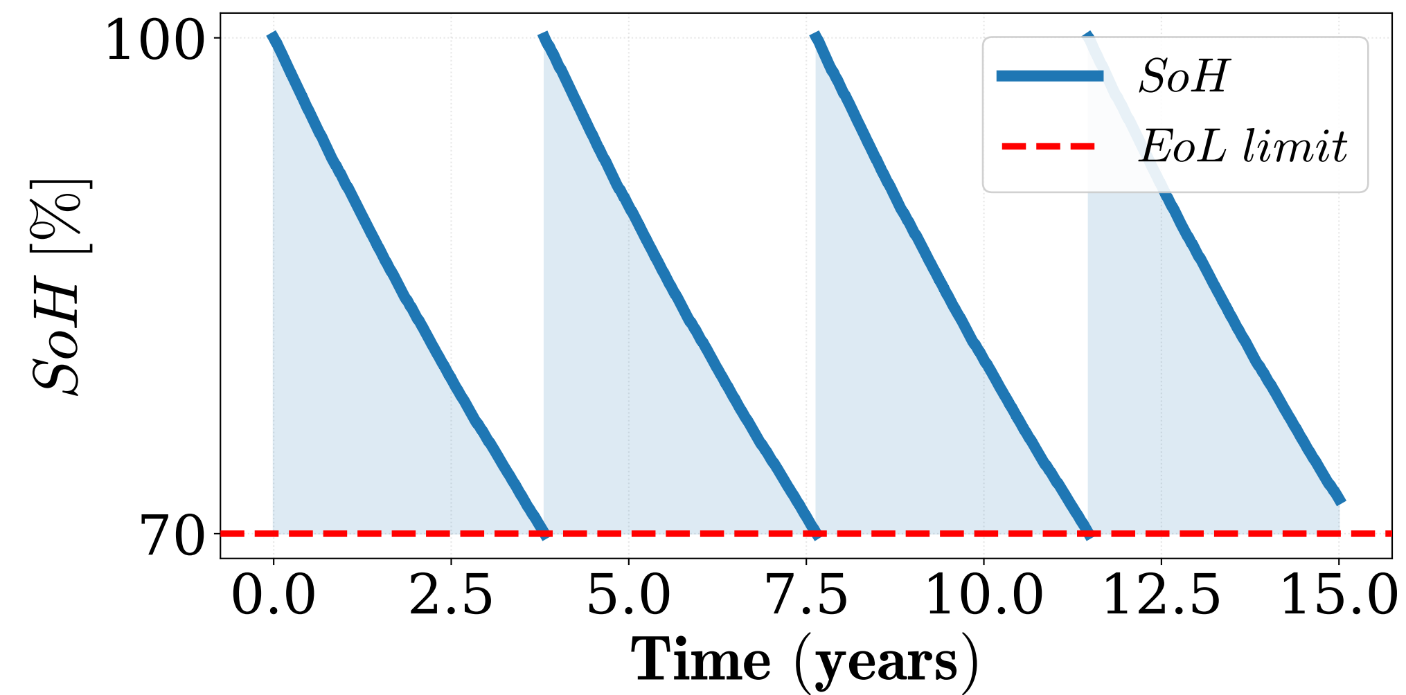
PEMFC Degradation
