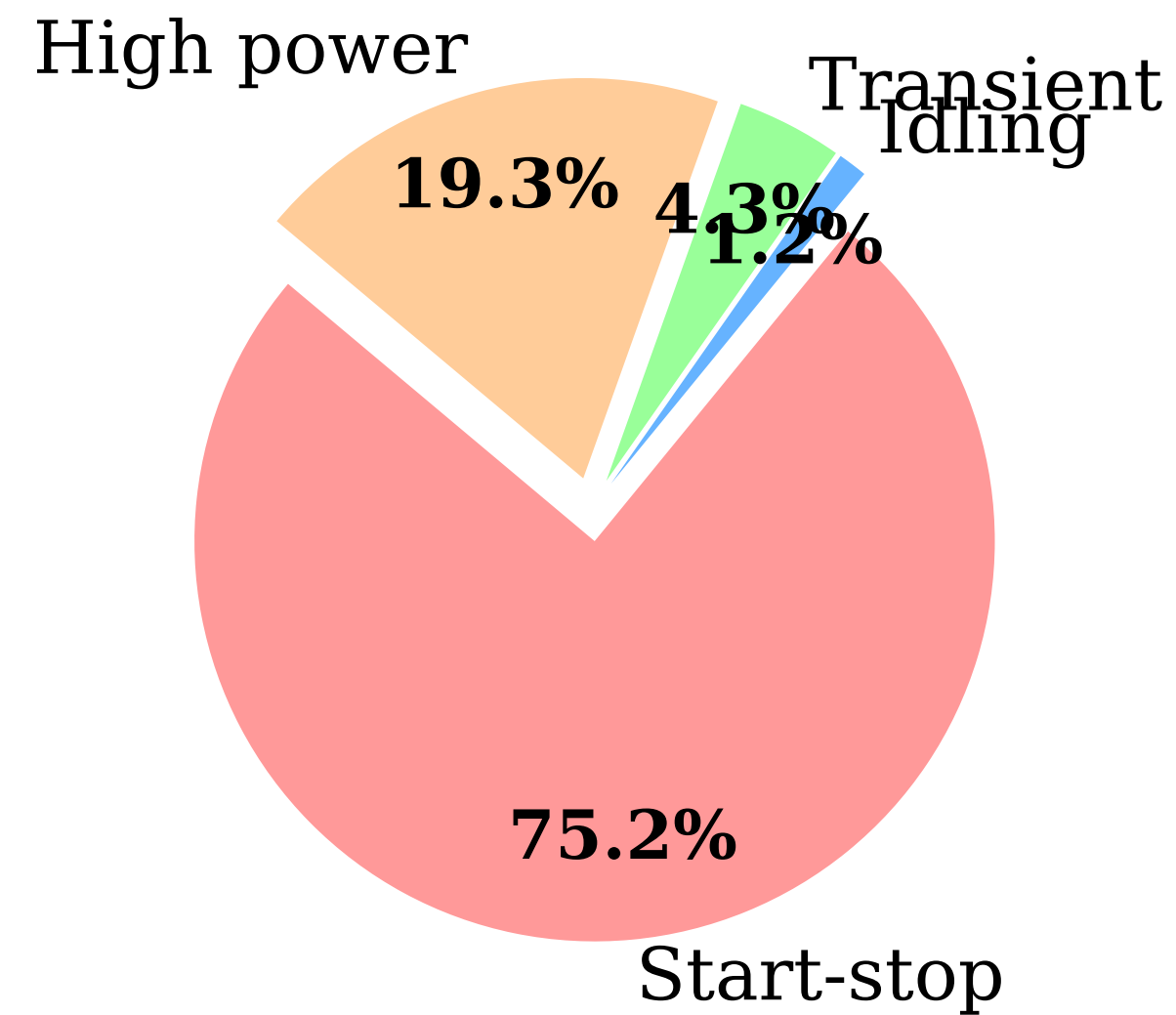
PEMFC Degradation
