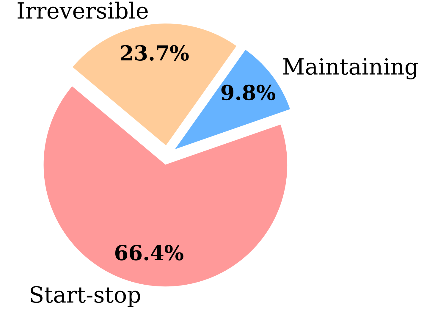
PEMWE Degradation
