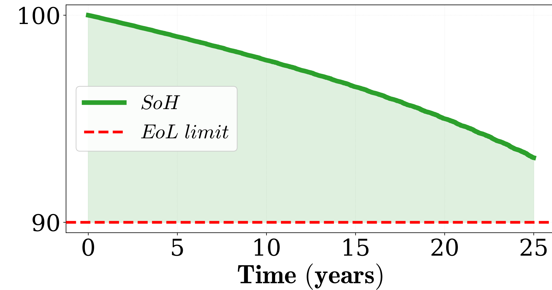
PEMWE Degradation
