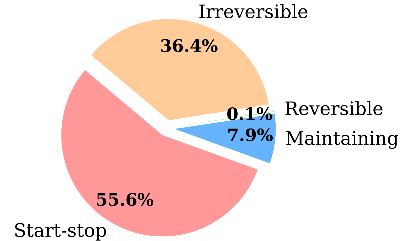
PEMWE Degradation
