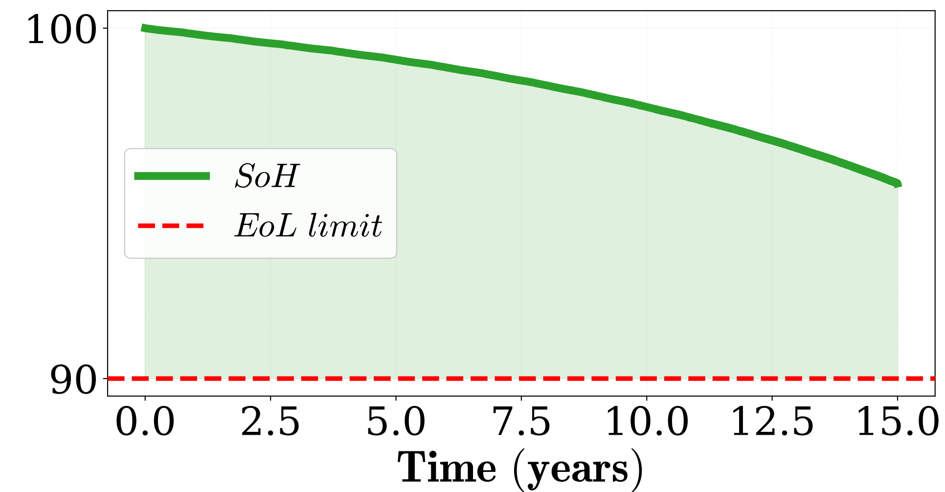
PEMWE Degradation
