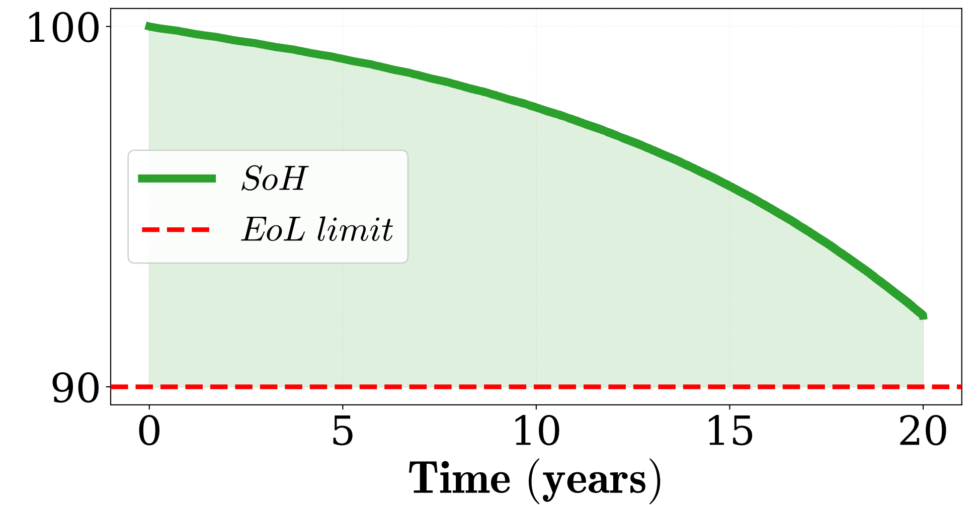
PEMWE Degradation
