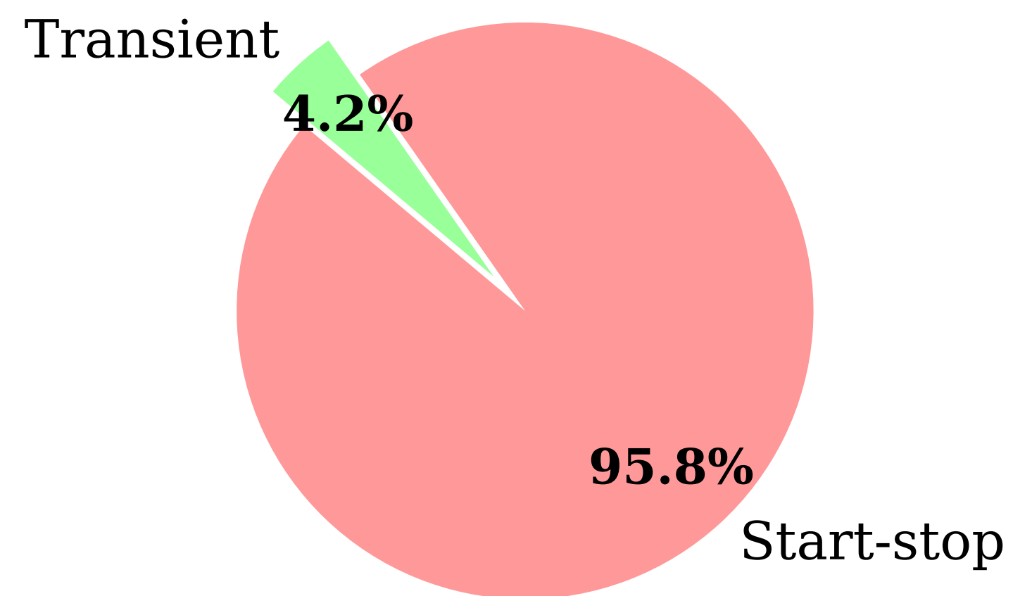
PEMFC Degradation
