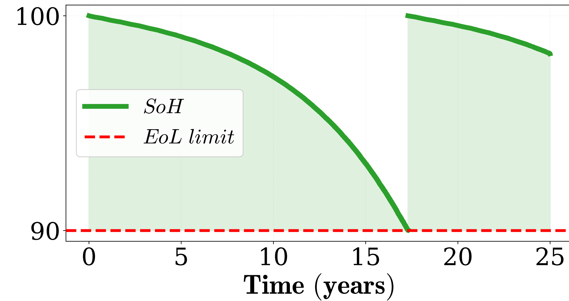
PEMWE Degradation
